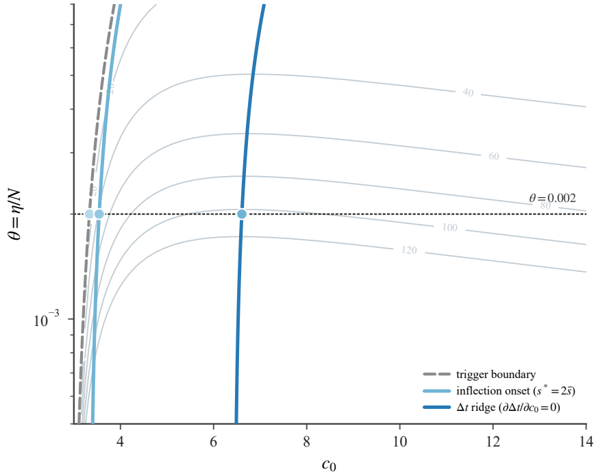
图 24: (\theta, c_0) 平面上的触发边界、内部拐点边界 s^* = 2\bar{s} 和控制持续时间驻点曲线 \partial \Delta t / \partial c_0 = 0 。灰色等值线表示控制持续时间, 水平点线为 \theta = 0.002 。
