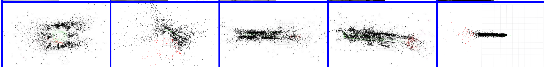
VINS- Fusion
