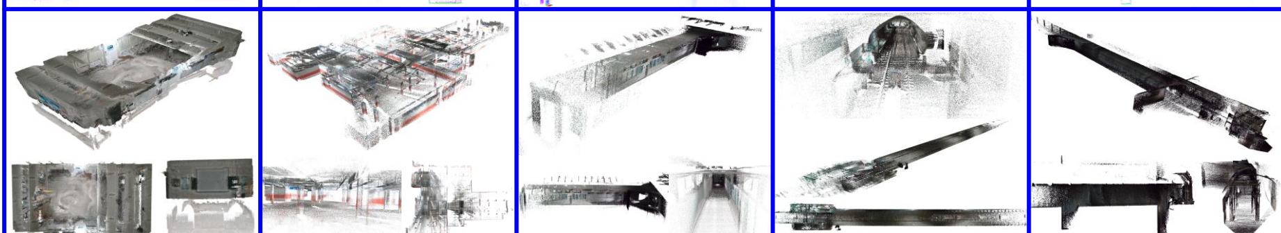
R 3 LIVE
