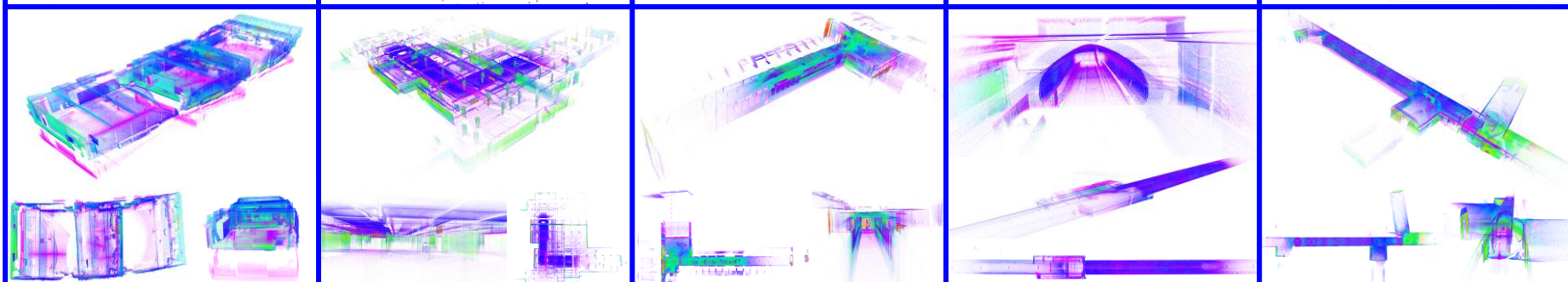
Fast- LIO2
