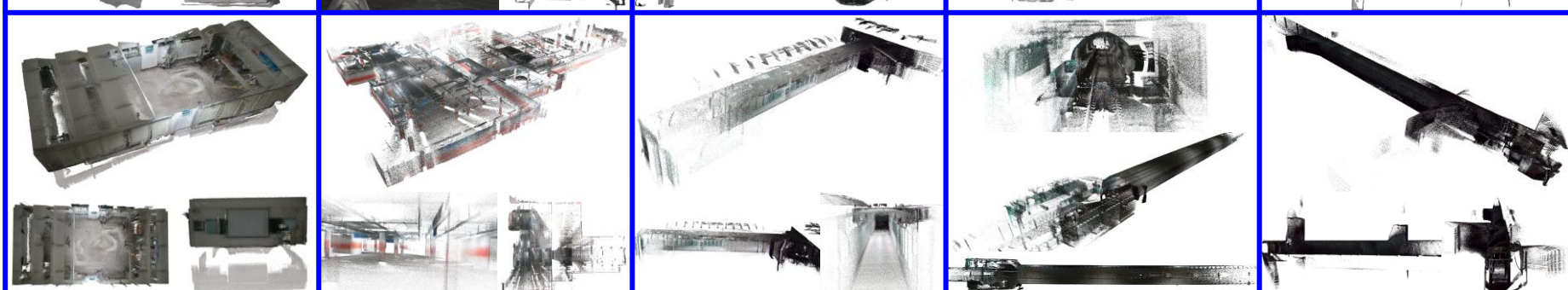
Fast- LIVO2
