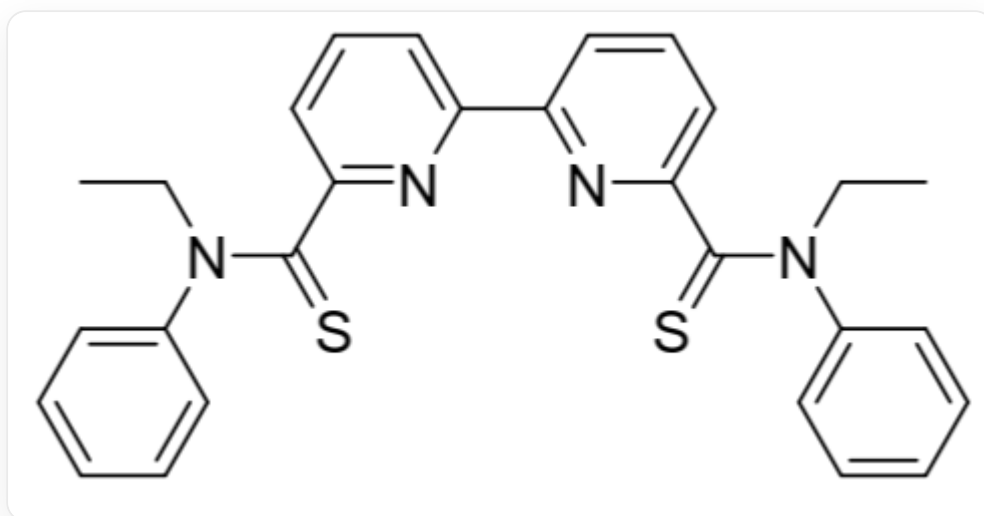
Fig .1, 图中分子以SMILES表示为:
