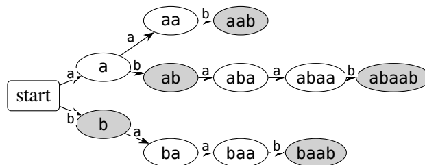
Hình 2: Trie hữu tố của S = abaab . Các nút tô xám ứng với các hữu tố của S .
