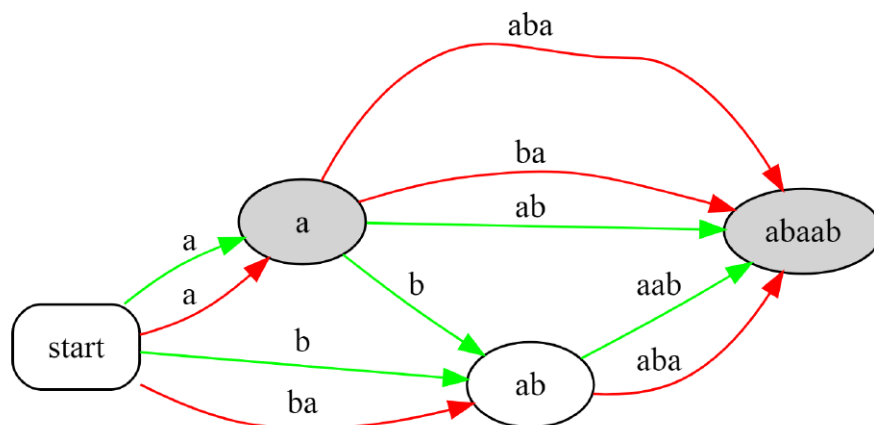
Hình ví dụ 5.1.3: suffix automaton nén đối xứng của S = abaab ; cạnh xanh là chuyển của xâu gốc, cạnh đỏ là chuyển của xâu đảo.
