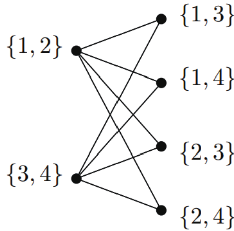
Hình 28: gán danh sách làm K_{2,4} không 2-choosable
