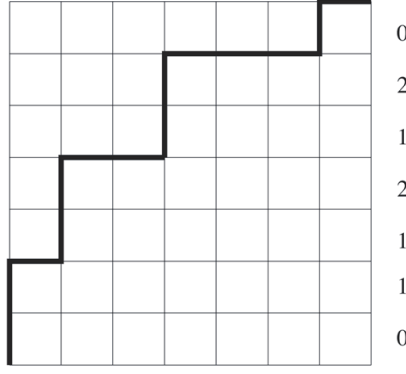
Hình 30: các giá trị a_i(\pi) trong area statistic
