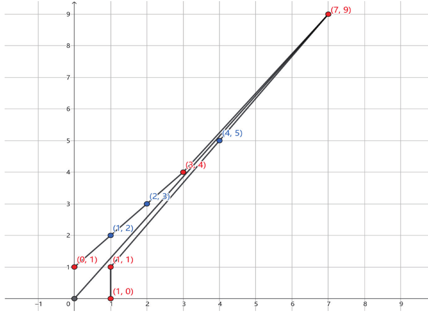
Hình 26: bao lồi của các hội tụ phân và phân số trung gian
