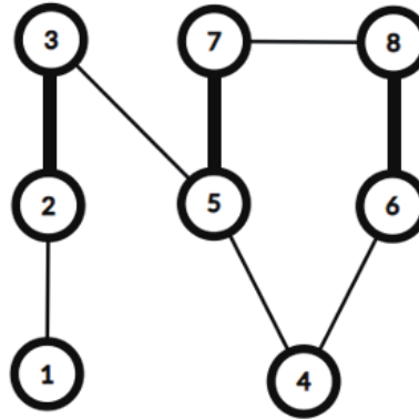
Hình 19: ví dụ BFS và bridge
