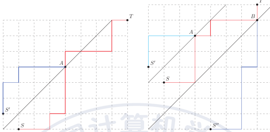
Hình 22: phản xạ với một biên và hai biên song song
