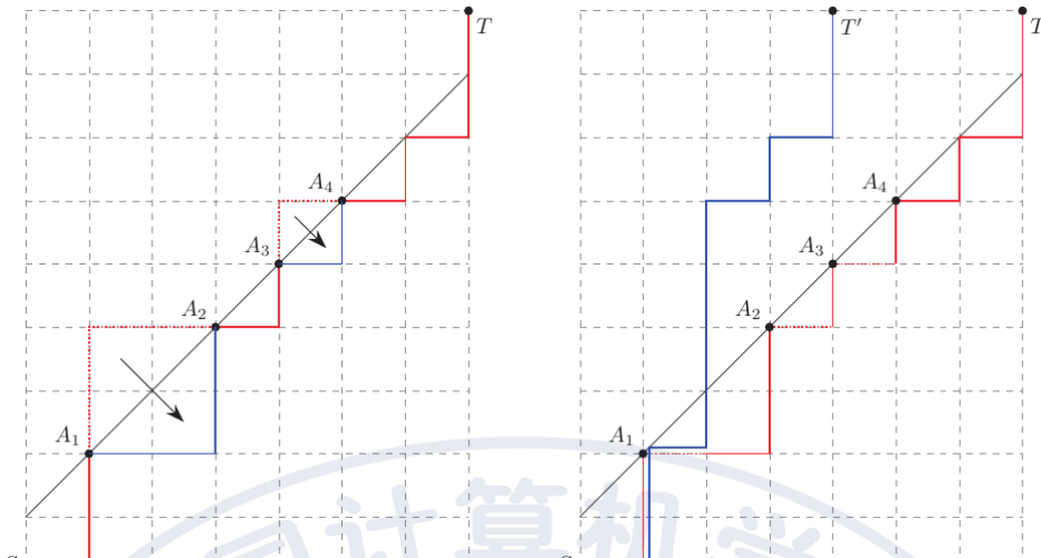
Hình 25: song ánh khi cố định số giao điểm với đường thẳng
