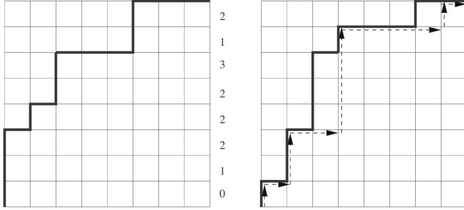
Hình 34: ví dụ song ánh \zeta biến \pi thành \pi'
