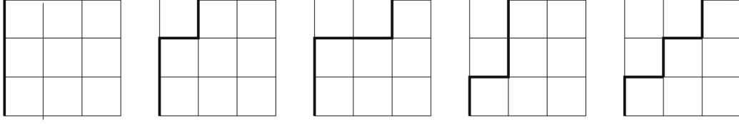
Hình 31: năm Dyck path khi n = 3 và area tương ứng
