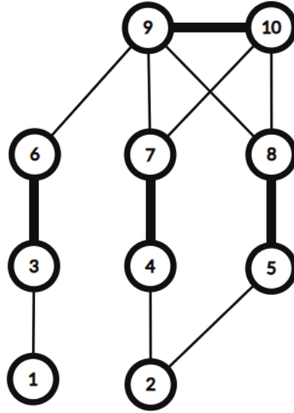
Hình 20: ví dụ chạy Bloss-Aug
