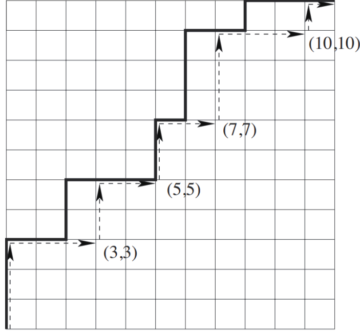
Hình 32: bounce path và các điểm chạm đường chéo
