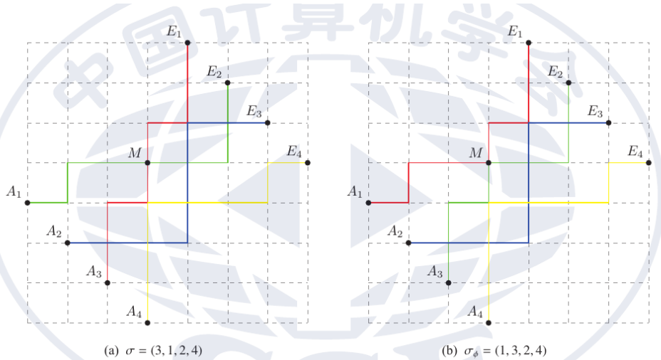
Hình 21: đối hợp đối dấu trong chứng minh LGV
