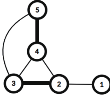
Hình 18: một ví dụ blossom
