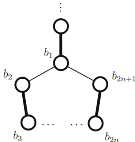
Hình 17: định nghĩa blossom và base
