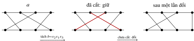
Hình 11: Minh họa phép nhân a \circ b trên biểu diễn dây của hoán vị. Tách b thành các đổi chỗ kề; với mỗi cặp dây, nếu chúng đã giao nhau trong a thì giữ nguyên, còn nếu chưa giao nhau thì thực hiện đổi chỗ.
