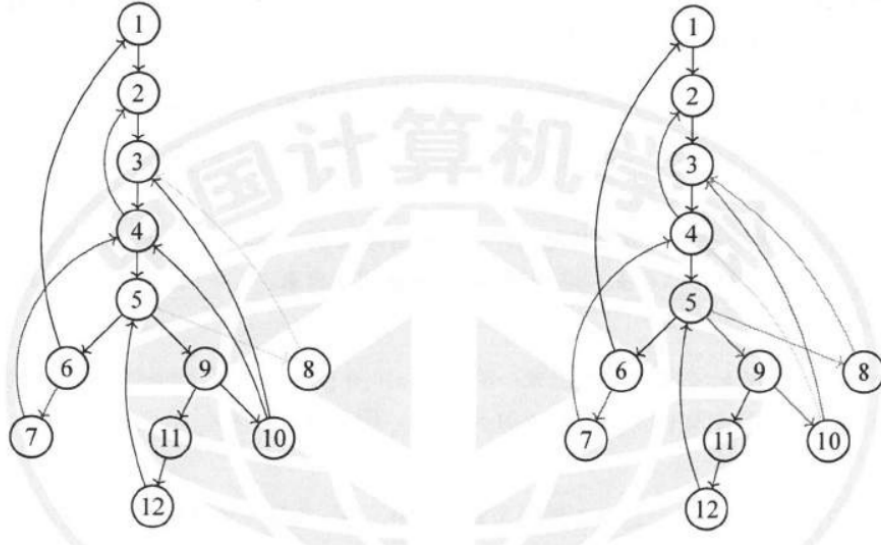
Hình 1: Ví dụ trong nguồn về các đoạn và các đường đi được chia từ cây DFS. Hai hình đặt cạnh nhau cho thấy cùng một đồ thị trước và sau khi các đường đi phân hoạch được làm nổi bật bằng những cung ngược.
