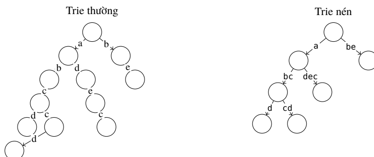
Hình 10: Trie thường và trie nén cho bốn xâu abcd, adec, abccd, be. Ở trie nén, các chuỗi bậc một như be, dec và cd được gộp thành nhãn cạnh.
