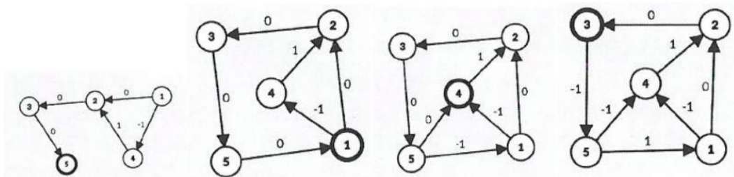
Hình 4: Sơ đồ trạng thái đá trong nguồn cho ví dụ Indiana Jones and the Uniform Cave . Đỉnh tô đậm là phòng hiện tại; nhãn 1, 0, -1 lần lượt biểu diễn đá đặt bên trái, bên phải và không đặt đá trên cạnh.
