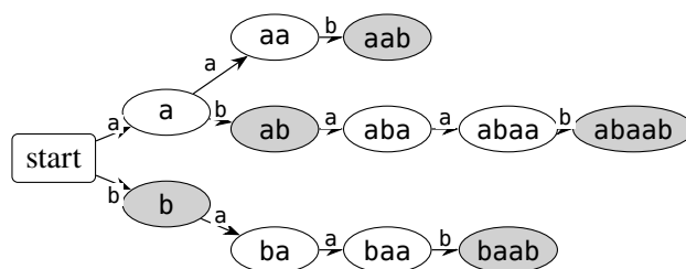
Hình 1: Trie hậu tố của S = \text{abaab} . Các nút tô xám ứng với các hậu tố của S .
