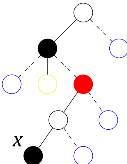
Hình 6: Các cây con cần cộng/trừ khi xử lý truy vấn trên đường từ x về gốc.
