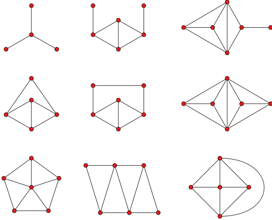
Hình 6: chín đồ thị cấm của Beineke
