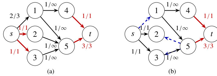
Hình 2: Ví dụ đồ thị hai phía trong nguồn: hình (a) minh họa cách chọn sai chỉ từ cạnh bão hòa; hình (b) cho thấy các đường dư màu xanh khiến cắt đúng phải lấy các cạnh đỏ phía đích.
