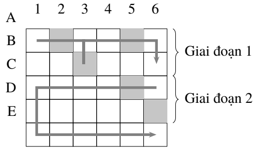
Hình 13: Chia thành các giai đoạn hai hàng: đi xuống hàng phụ rồi quay lại giữ nguyên chỗ lẻ của đường đi chính.
