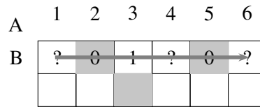
Hình 14: Chuỗi yêu cầu 0, 1, ? trên một giai đoạn: 0 là vào ô ở giây chẵn, 1 là vào ô giây lẻ để lấy viên ở hàng dưới, còn ? có thể gắn để nối hai phía.
