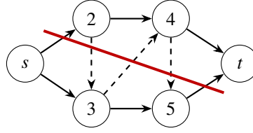
Hình 1: Ví dụ cắt nhỏ nhất trong nguồn: các đỉnh dưới đường đỏ thuộc S ; các đỉnh còn lại thuộc T .
