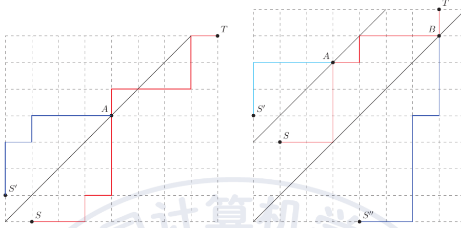
Hình 19: phản xạ với một biên và hai biên song song
