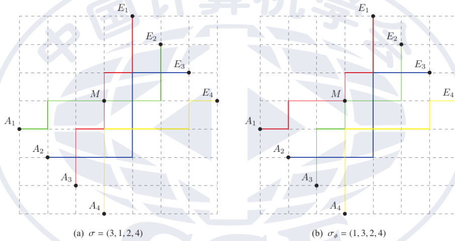
Hình 18: đối hợp đối dấu trong chứng minh LGV
