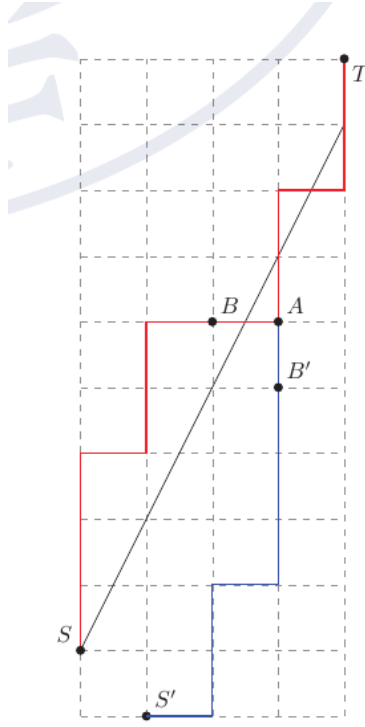
Hình 20: phương pháp quay
