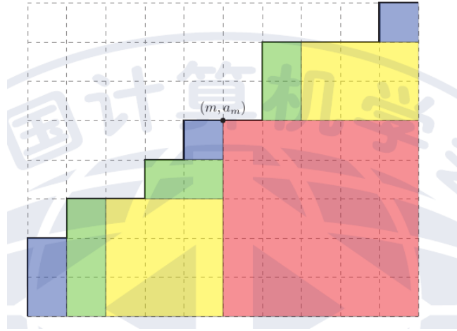
Hình 21: lưới bậc thang trong chia để trị
