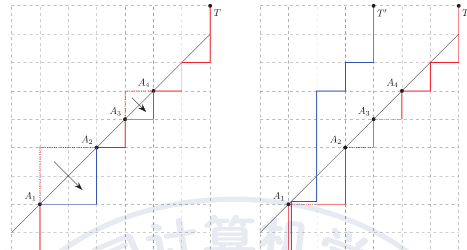
Hình 22: song ánh khi cố định số giao điểm với đường thẳng
