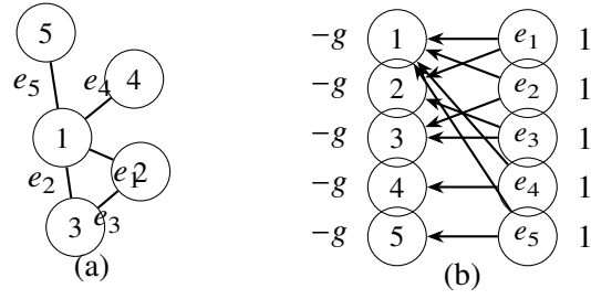
Hình 6: Thuật toán sơ bộ cho đồ thị con mật độ lớn nhất: mỗi cạnh của G trở thành một đỉnh trọng số 1 trong đồ thị đóng.
