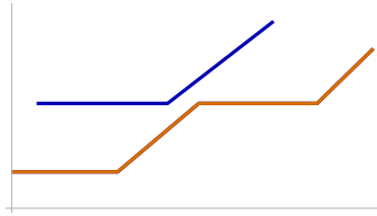
Bao dưới có thể sinh nhiều đoạn gấp khúc.
