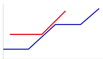
Lấy bao trên của hai nhãn lịch sử.
