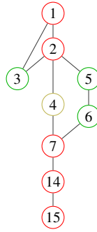
Phân loại đỉnh trên đường từ 15 tới 1.
