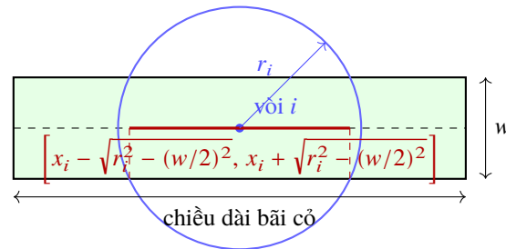
Hình 4.1: mặt cắt bãi cỏ; vòng tròn tưới của một vòi cắt mép bãi thành một đoạn hữu ích trên chiều dài.
