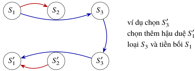
Hình 4: Các cung đỏ và xanh là hai chuỗi đối xứng. Chọn một thành phần sẽ chọn các hậu duệ của nó và loại thành phần đối ứng cùng các tiền bối.
