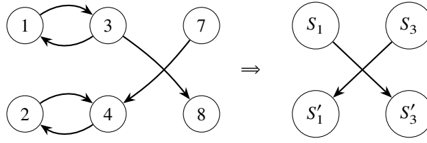
Hình 2: Co hai chu trình \{1, 3\} và \{2, 4\} thành hai thành phần đối ứng S_1, S'_1 ; các cung giữa thành phần tạo thành một DAG.
