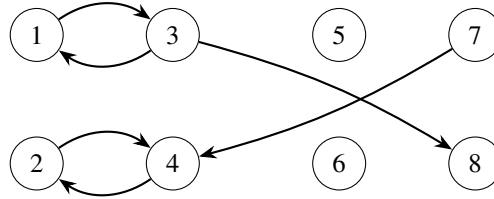
Hình 1: Đồ thị kéo theo của ví dụ bốn nhóm: chọn 1 kéo theo 3, rồi kéo theo 8; do đó 2, 4, 7 bị loại, còn 5, 6 chưa bị quyết định.
