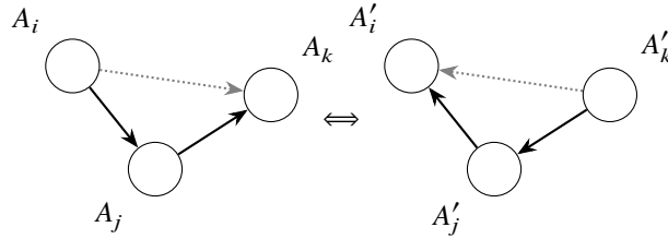
Hình 3: Đối xứng truyền: nếu A_i \rightarrow^* A_k qua một chuỗi kéo theo, thì chuỗi đối ứng A'_k \rightarrow^* A'_i cũng tồn tại.
