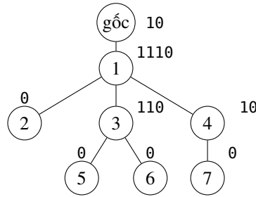
Hình 11: Một cây và mã của từng đỉnh.
