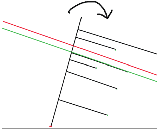
Hình 3: đường quét xoay và các thời điểm đổi thứ tự hình chiếu
