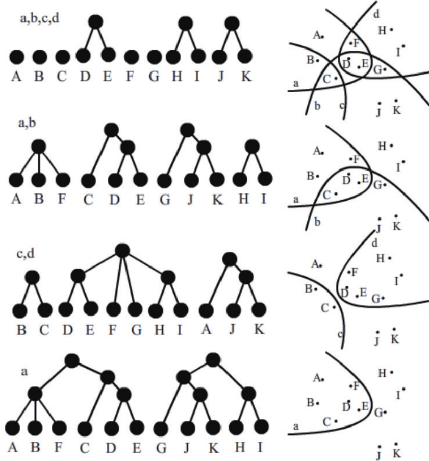
Hình 2: các trạng thái rừng có gốc khi chuyển giữa các quan hệ tương đương
