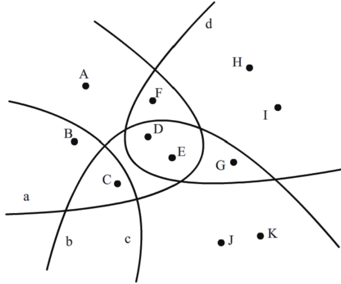
Hình 1: các đường cong chia điểm thành các lớp tương đương
