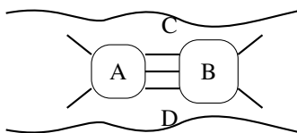
Hình 1: sơ đồ bảy cây cầu Königsberg trong nguồn.
