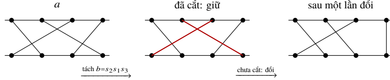
Hình 12: Minh họa phép nhân a \circ b trên biểu diễn dây của hoán vị. Tách b thành các đối chố kề; với mỗi cặp dây, nếu chúng đã giao nhau trong a thì giữ nguyên, còn nếu chưa giao nhau thì thực hiện đổi chỗ.
