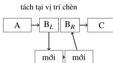
Figure 1: Chèn trong danh sách khối: tách khối hiện tại và nối các khối mới vào giữa.
