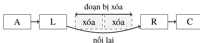
Figure 2: Xóa trong danh sách khối: sau khi tách hai biên, bỏ các khối ở giữa và nối lại.
