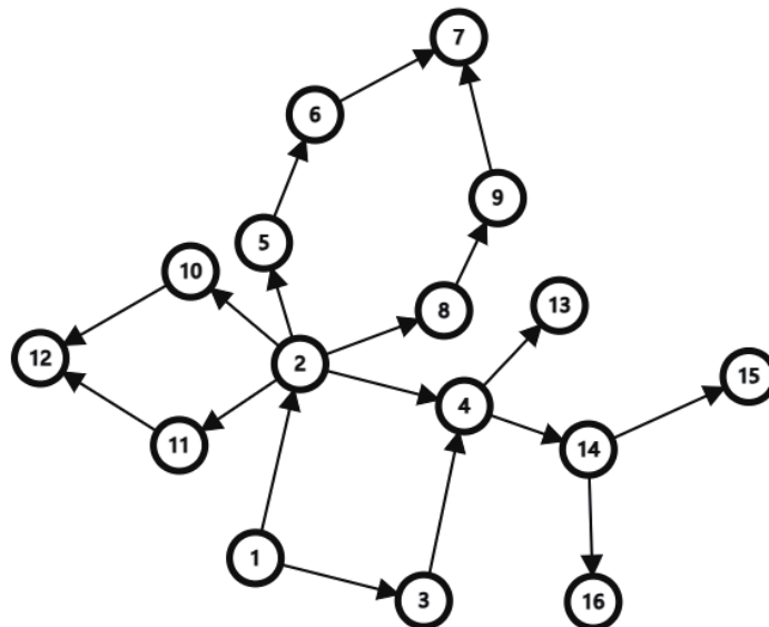
Hình 8: một cactus cạnh hướng ra lá
