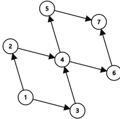
Hình 7: ví dụ cho thấy cách gộp trực tiếp không còn đúng
