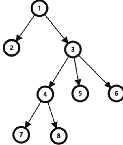
Hình 6: ví dụ cây hướng ra lá
