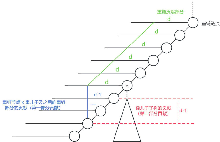
Hình 11: ba vùng đóng góp quanh một đoạn chuỗi nặng
