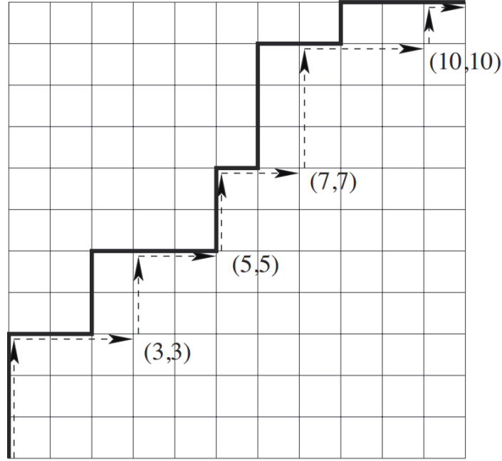
Hình 25: bounce path và các điểm chạm đường chéo
