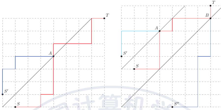
Hình 15: phản xạ với một biên và hai biên song song
