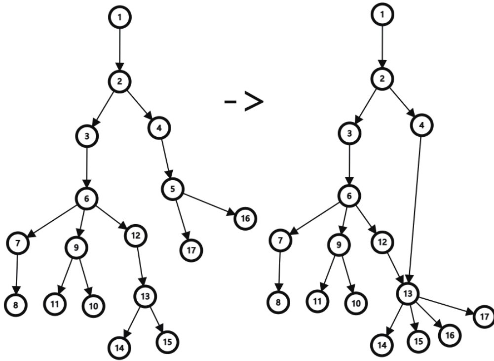
Hình 9: điều chỉnh đồ thị khi u = 13 và v = 5
