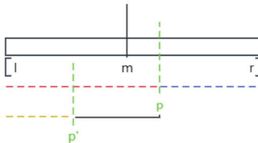
Hình 13: chia cụm theo trung vị có trọng số
