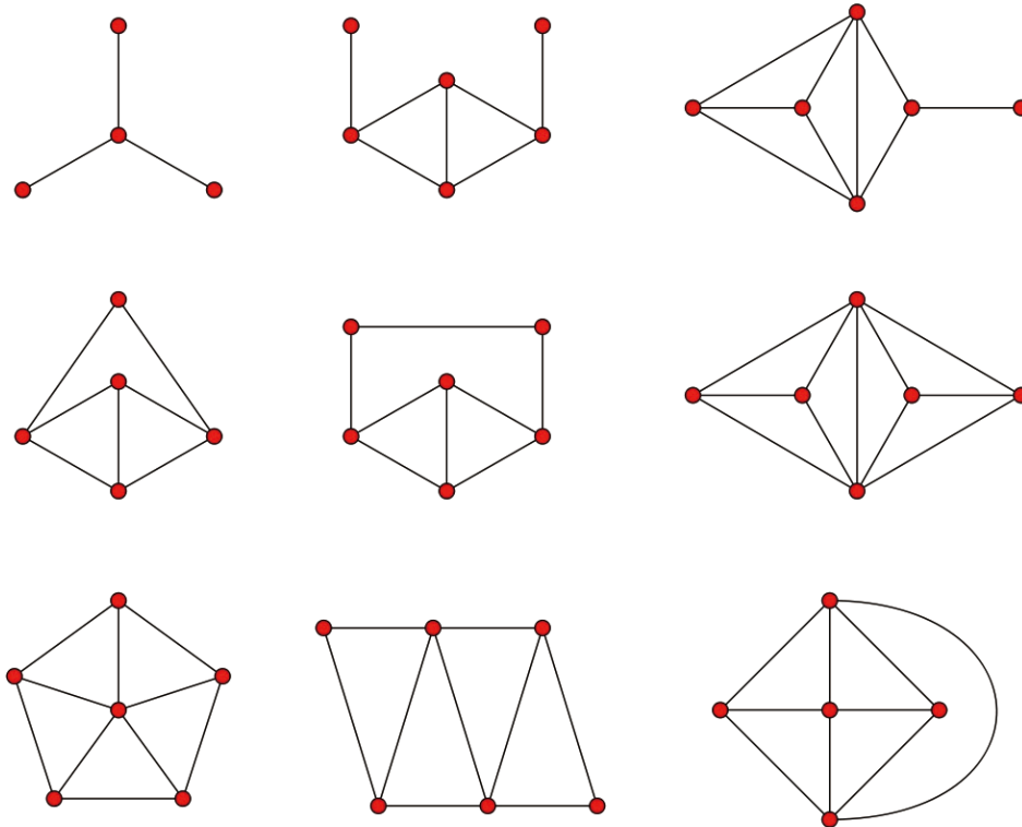
Hình 10: chín đồ thị cấm của Beineke
