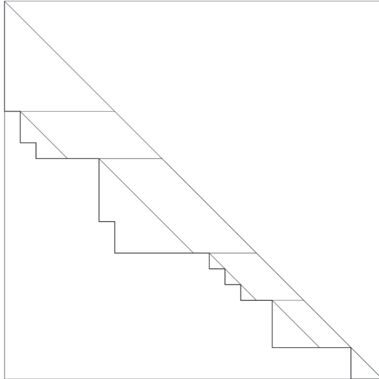
Hình 28: miền con trong chứng minh q -functional composition
