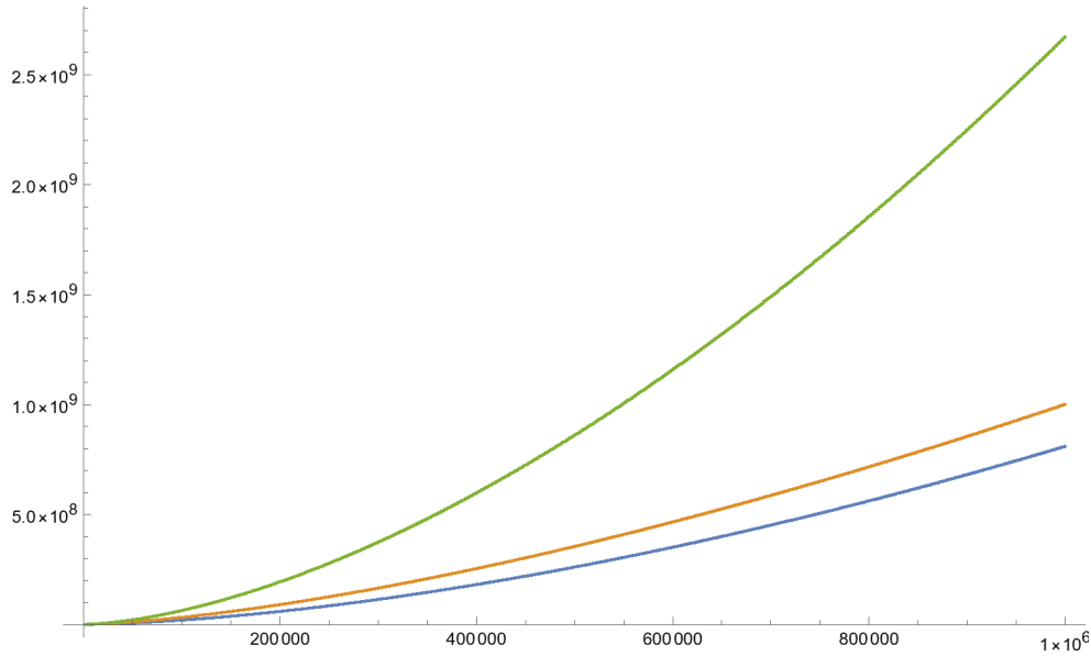
Hình 20: số lần sửa trong Dynamic-gcd so với đường chuẩn x\sqrt{x}
