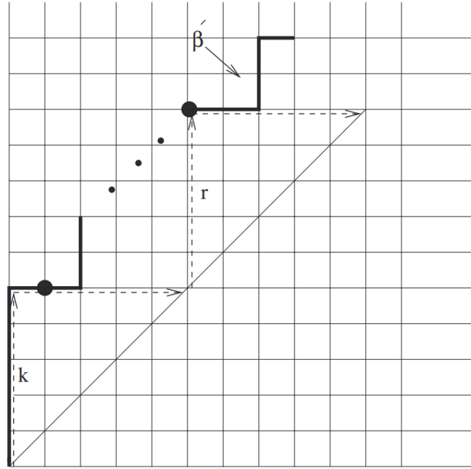
Hình 26: chia \beta theo hai lần bật đầu và dựng \beta'
