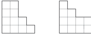
Hình 22: Ferrers graph của (4, 3, 2, 2) và conjugate partition
