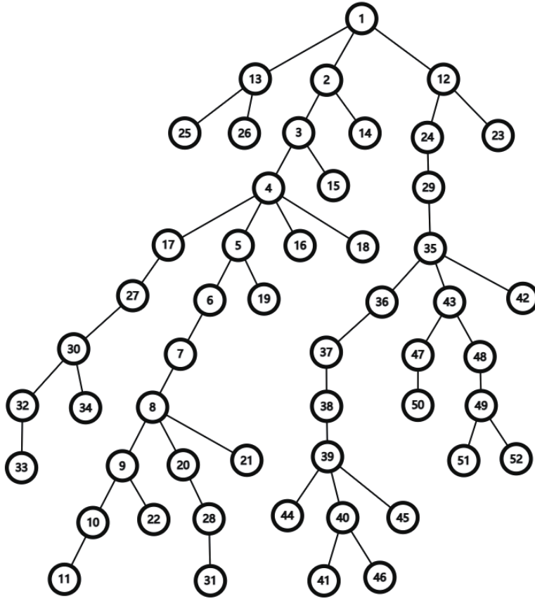
Hình 12: một cách đánh nhãn hợp lệ theo quy tắc duyệt chuỗi nặng
