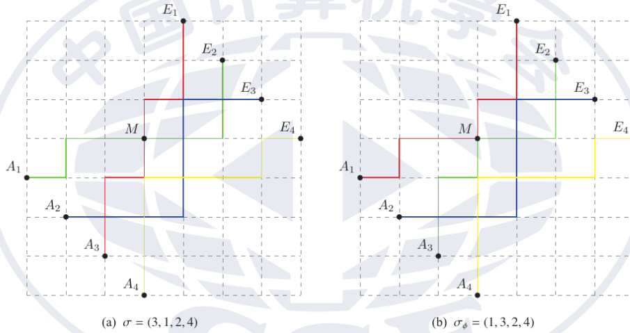
Hình 17: đối hợp đối dấu trong chứng minh LGV
