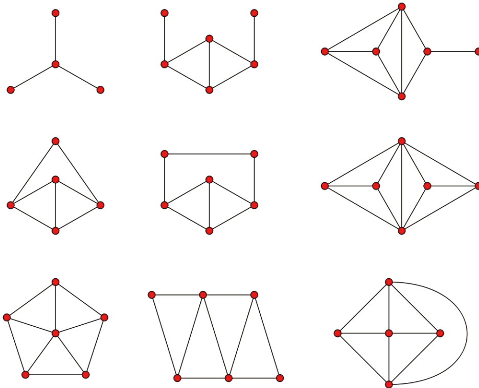
Hình 13: chín đồ thị cấm của Beineke
