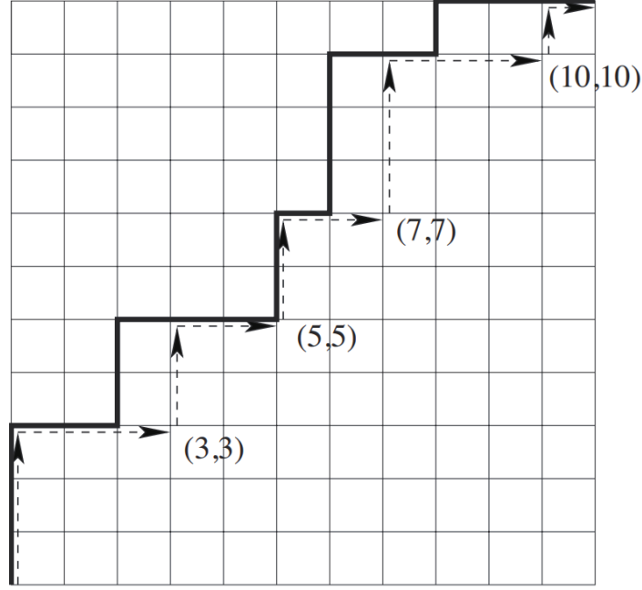
Hình 28: bounce path và các điểm chạm đường chéo
