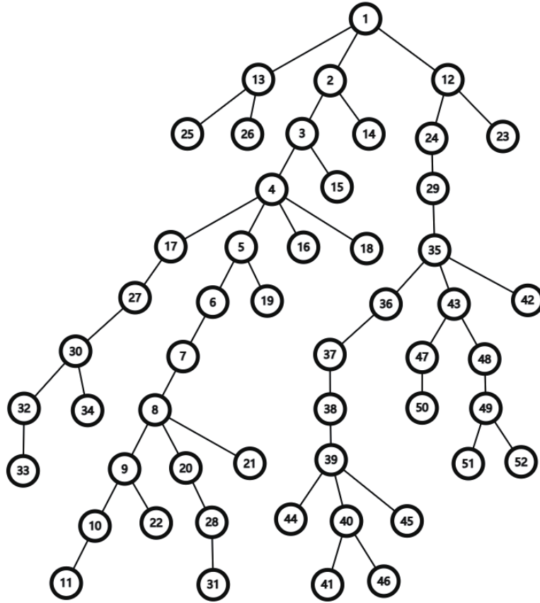
Hình 15: một cách đánh nhãn hợp lệ theo quy tắc duyệt chuỗi nặng
