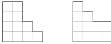
Hình 25: Ferrers graph của (4, 3, 2, 2) và conjugate partition
