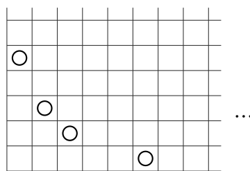
Vị trí trong Nim hai chiều.
