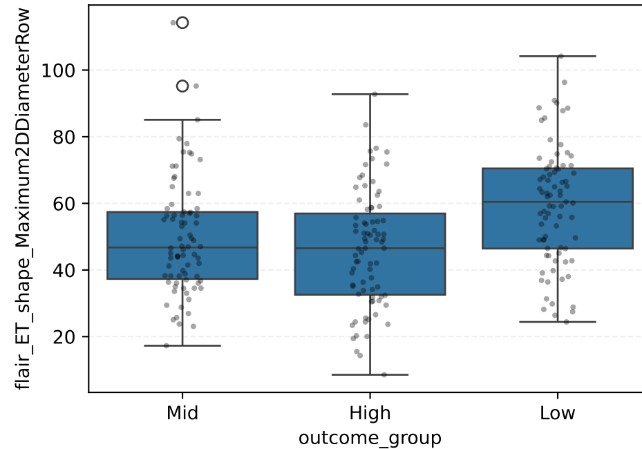
flair_ET_shape_Maximum2DDiameterRow
