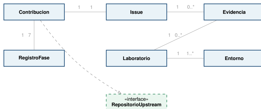
Figura 34: Clases de diseño, relaciones y multiplicidades. Contribucion depende de la interfaz RepositorioUpstream, no de su implementación.
