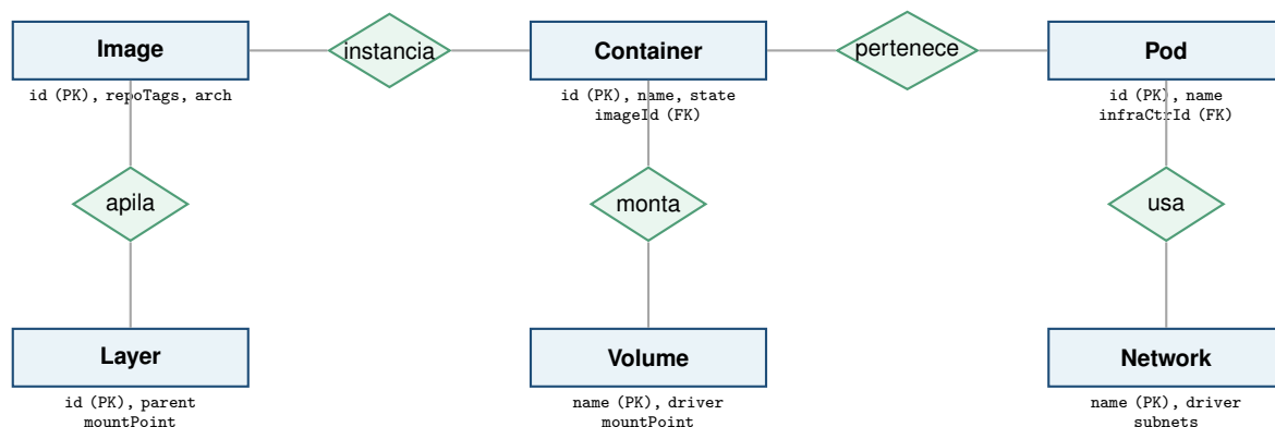
Figura 17: Esquema relacional equivalente al estado persistido por libpod y containers/storage.
