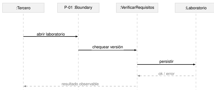
Figura 33: Diagrama de secuencia de CU-001-006 — Reproducción por tercero.
