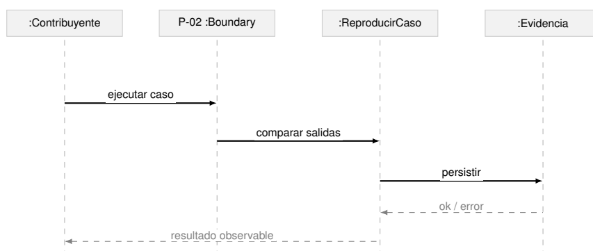
Figura 30: Diagrama de secuencia de CU-001-003 — Reproducción.
