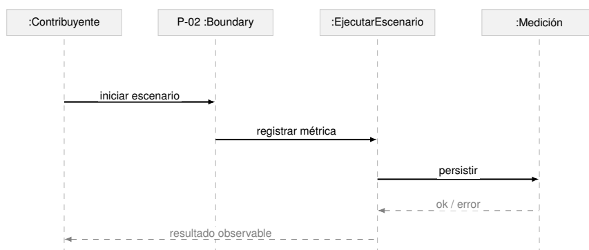
Figura 32: Diagrama de secuencia de CU-001-005 — Escenario de evaluación.
