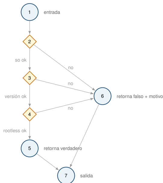
Figura 35: Grafo de flujo de control de requisitosCumplidos . Nodos 2, 3 y 4 son decisiones; aristas: 9; nodos: 7.
