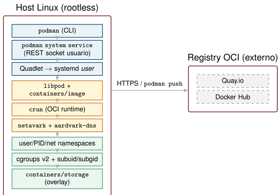
Figura 18: Despliegue de Podman rootless sobre un host Linux: userspace (CLI, service , Quadlet), runtime (libpod, crun, networking) y soporte del kernel (namespaces, cgroups v2, storage). Caso testigo PR #28637 ejerce la flecha hacia el registry .
