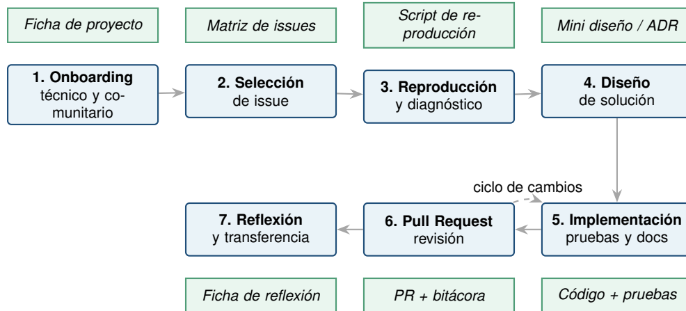
Figura 6: Mapa de las siete fases del marco metodológico, con sus artefactos verificables. Adaptado de [7].
