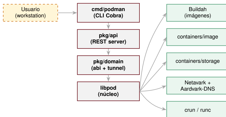
Figura 15: Componentes principales del ecosistema Podman: cadena interna (CLI → API → dominio → libpod) y dependencias del núcleo sobre el resto del proyecto containers/. Adaptado de [6, 3].
