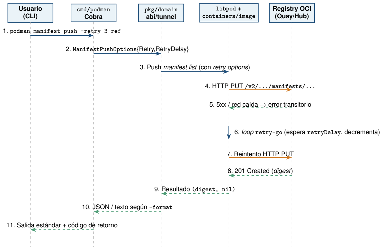
Figura 13: Diagrama de secuencia del comando podman manifest push -retry . Atraviesa CLI (Cobra), capa de dominio, núcleo libpod/containers/image y registry OCI. Caso testigo del flujo: PR #28637.
