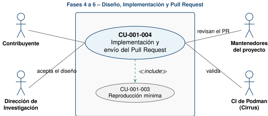
Figura 10: CU-001-004 – Implementación y envío de un Pull Request al proyecto Podman.
