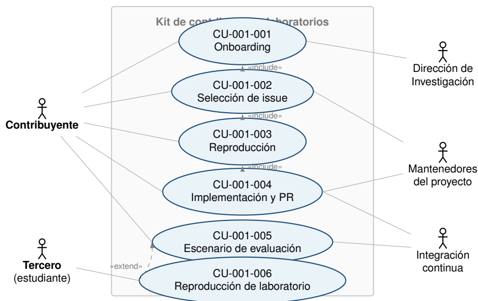
Figura 19: Diagrama general de casos de uso con límite del sistema, actores primarios (izquierda) y secundarios (derecha).
