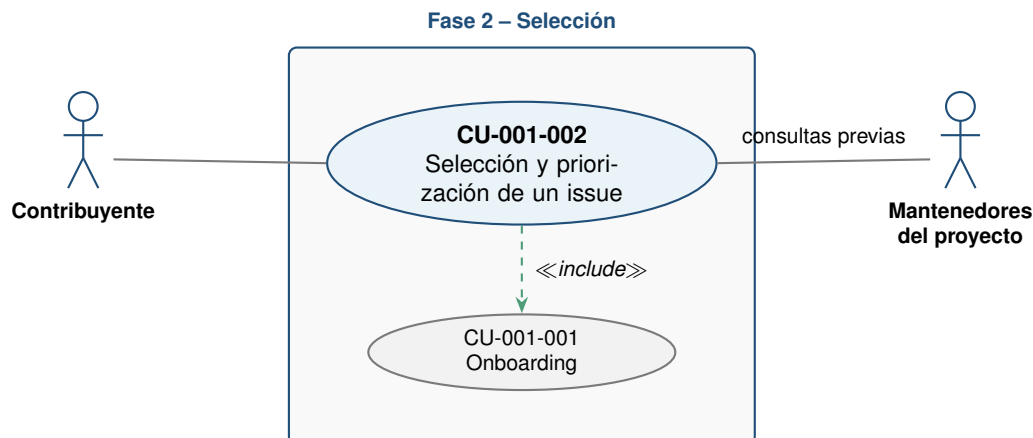
Figura 8: CU-001-002 – Selección y priorización de un issue para contribuir.
