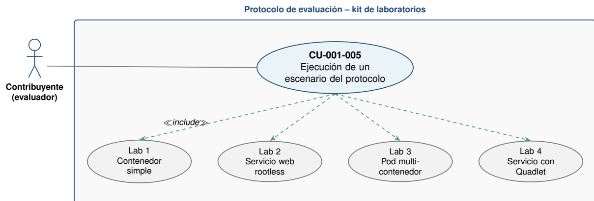
Figura 11: CU-001-005 – Ejecución de un escenario del protocolo de evaluación. Los cuatro laboratorios del kit son casos incluidos.
