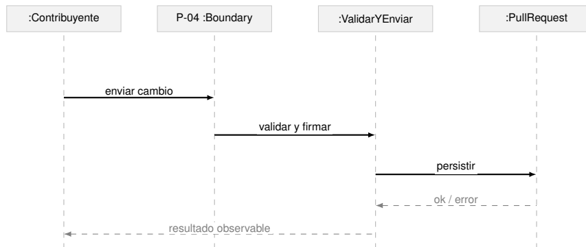
Figura 31: Diagrama de secuencia de CU-001-004 — Implementación y PR.
