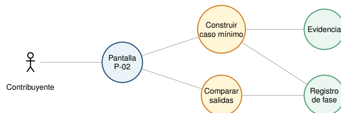
Figura 24: Diagrama de robustez de CU-001-003 — Reproducción.
