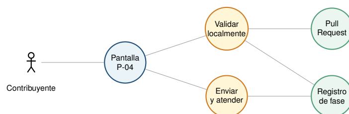
Figura 25: Diagrama de robustez de CU-001-004 — Implementación y PR.
