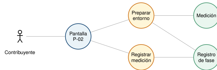
Figura 26: Diagrama de robustez de CU-001-005 — Escenario de evaluación.
