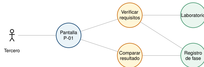
Figura 27: Diagrama de robustez de CU-001-006 — Reproducción por tercero.
