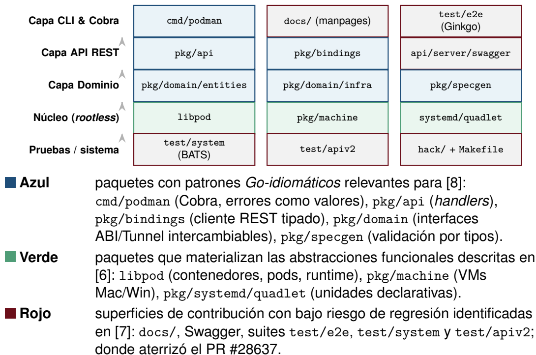
Figura 14: Diagrama de paquetes de containers/podman agrupado por capa. La flecha lateral indica el flujo principal de invocación CLI → API → Dominio → Núcleo → Pruebas.
