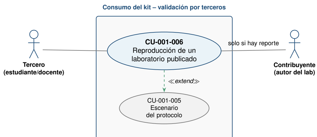
Figura 12: CU-001-006 – Reproducción de un laboratorio publicado por un tercero.
