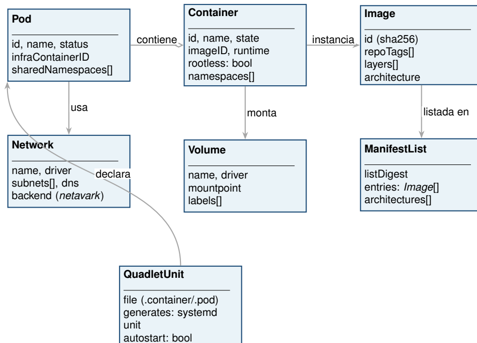
Figura 16: Modelo de dominio de Podman: Pod, Container, Image, ManifestList, Network, Volume y QuadletUnit, con sus relaciones principales. Tomado del análisis sobre commit 9f02e222.
