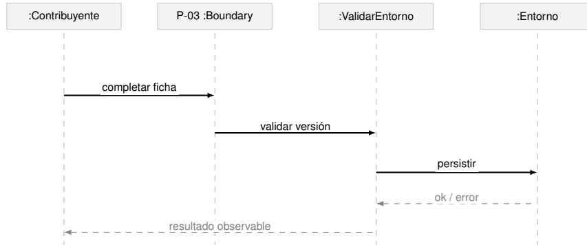
Figura 28: Diagrama de secuencia de CU-001-001 — Onboarding.
