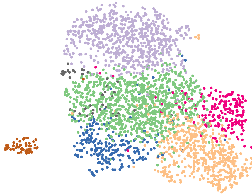
Louvain
