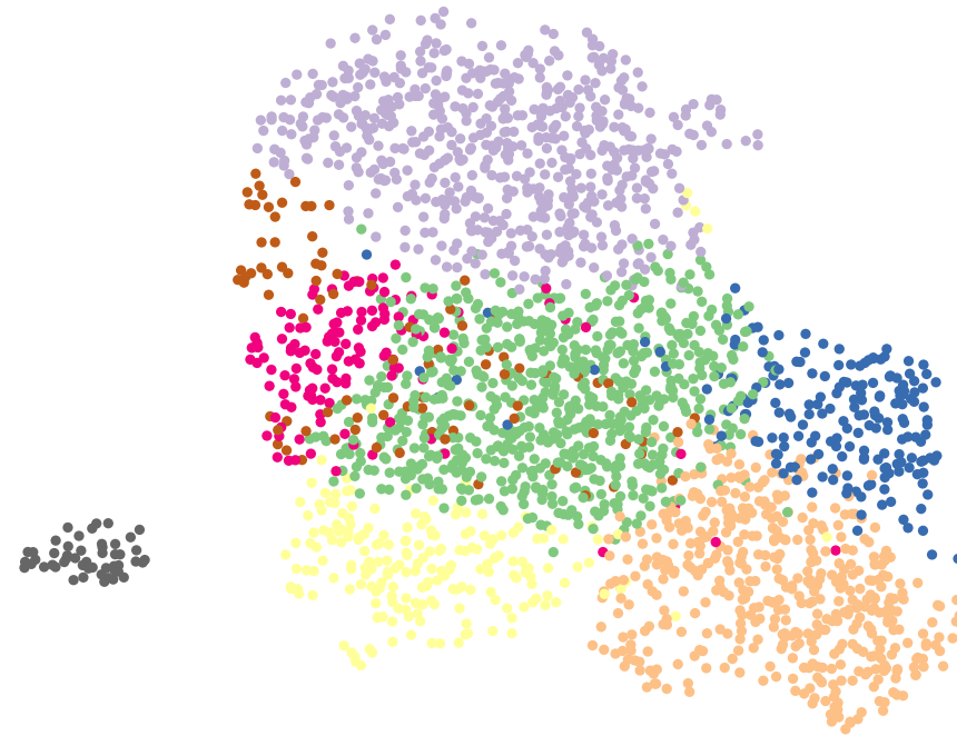
Leiden
