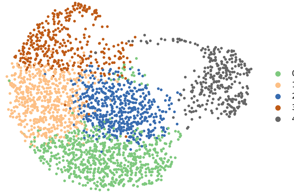
Louvain
