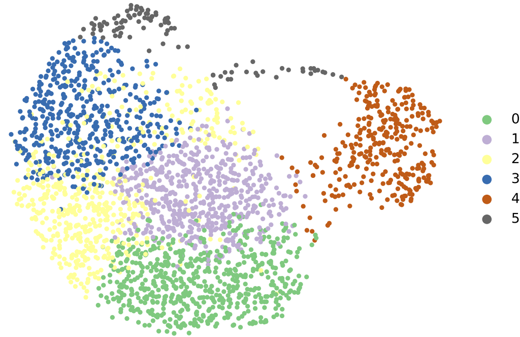
Leiden
