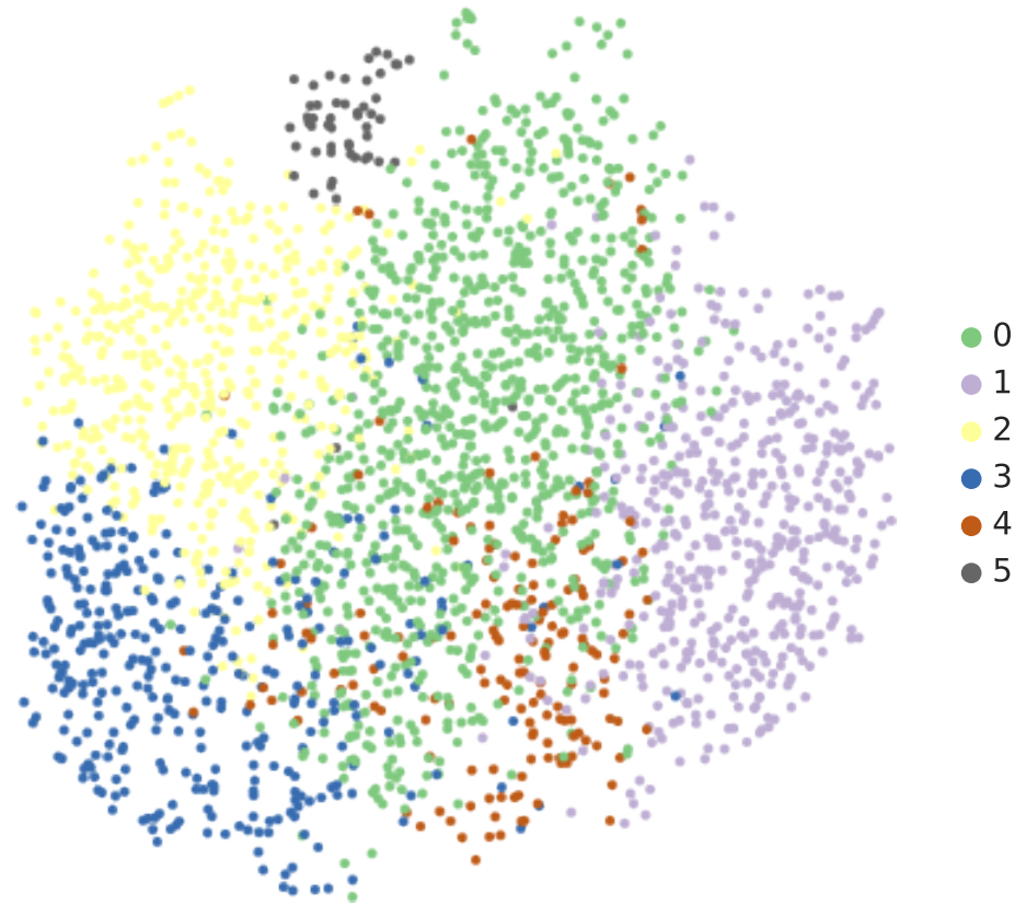
Louvain
