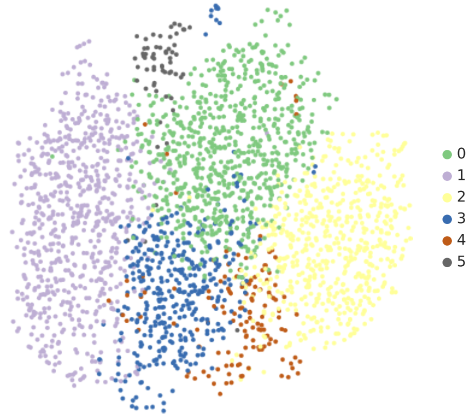
Leiden
