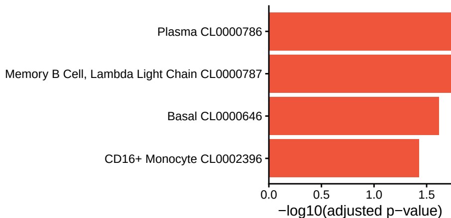
cluster_2
