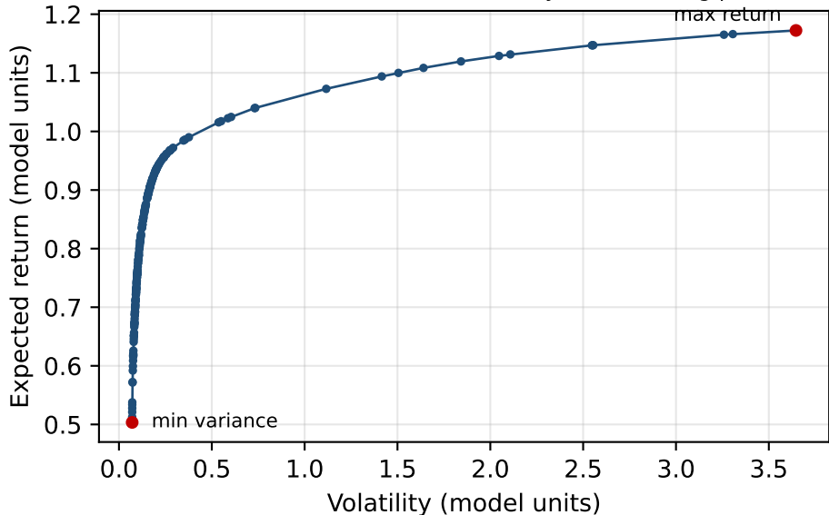
Efficient frontier: 200 assets, 2000 days (202 turning points)
