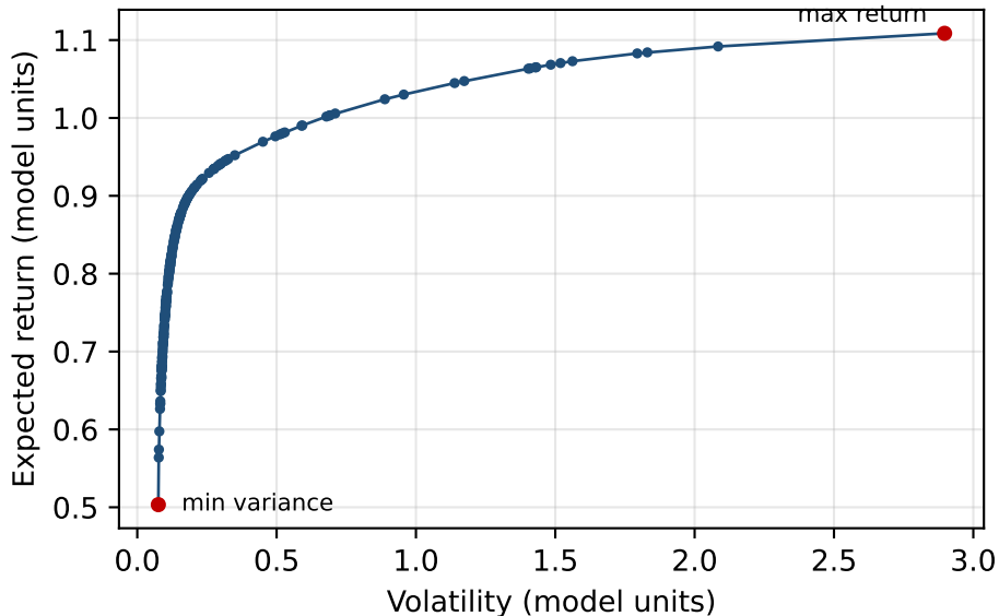
Efficient frontier: 200 assets, 2000 days (207 turning points)
