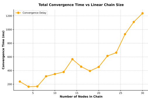
FIGURE 21 – Temps de convergence de la topologie dans une chaîne linéaire de nœuds.
