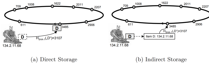
FIGURE 8 – Comparaison entre stockage direct et stockage indirect. [Source:schéma pris des notes de cours DBLP:conf/p2p/WehrleGR05 ]
