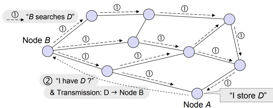
FIGURE 3 – Flooding Search : diffusion récursive de requêtes, puis retour des nœuds ayant la donnée. [Source:schéma pris des notes de cours DBLP:conf/p2p/WehrleGR05 ]
