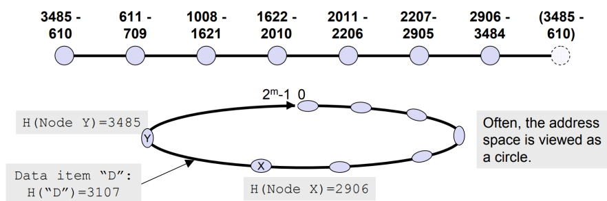
FIGURE 6 – Espace d'adressage linéaire partitionné entre pairs. [Source:schéma pris des notes de cours DBLP:conf/p2p/WehrleGR05 ]
