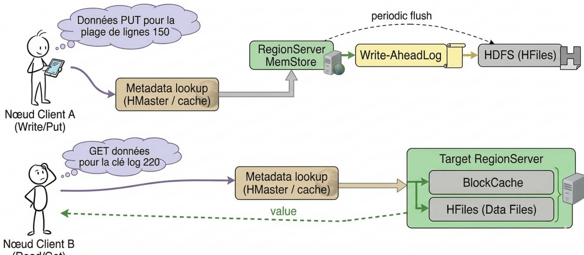
FIGURE 10 – Diagramme simplifié des flux PUT/GET dans HBase. Pour un PUT (client A), le client commence par une résolution de métadonnées (HMaster/cache), envoie l'écriture au RegionServer ciblé (MemStore), puis la donnée est sécurisée via le Write-Ahead Log avant d'être persistée sous forme de HFiles sur HDFS (flush périodique). Pour un GET (client B), le client résout d'abord la localisation de la région, interroge le RegionServer cible, puis la valeur est servie depuis le BlockCache ou les HFiles selon la disponibilité des blocs. Cette vue fournit une lecture opérationnelle concise des chemins d'écriture et de lecture dans HBase.
