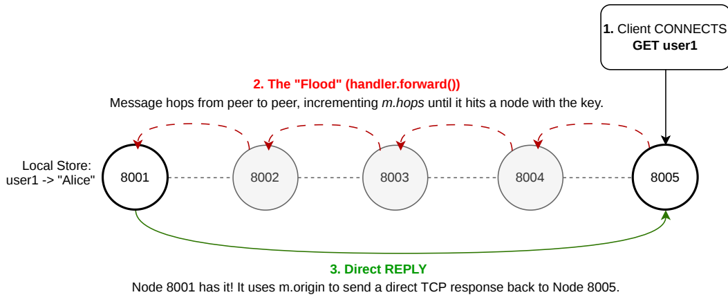
FIGURE 13 – Recherche par inondation dans l'approche naïve. Le nœud 8005 émet une requête GET user1 ; celle-ci est relayée de proche en proche par les pairs intermédiaires, avec incrément du compteur de sauts, jusqu'au nœud 8001 qui possède la donnée dans son stockage local. Dans ce sens, le flooding corrige partiellement les erreurs de placement ou de vue locale : même si le demandeur ne connaît pas le bon propriétaire, la propagation augmente ses chances d'atteindre le nœud qui détient effectivement la donnée.
