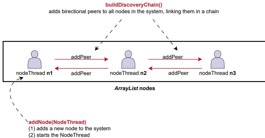
FIGURE 14 – Topologie et initialisation du réseau via DHTSystem. Ce schéma illustre l'organisation des nœuds stockés dans une ArrayList. En bas, la fonction addNode() est indiquée comme responsable de l'ajout d'un nouveau nœud et du démarrage de son thread. En haut, la fonction buildDiscoveryChain() est mise en évidence : elle parcourt la liste pour établir des connexions bidirectionnelles entre les nœuds voisins. Ces connexions sont matérialisées par les flèches rouges addPeer , transformant la simple liste en une chaîne de propagation opérationnelle.
