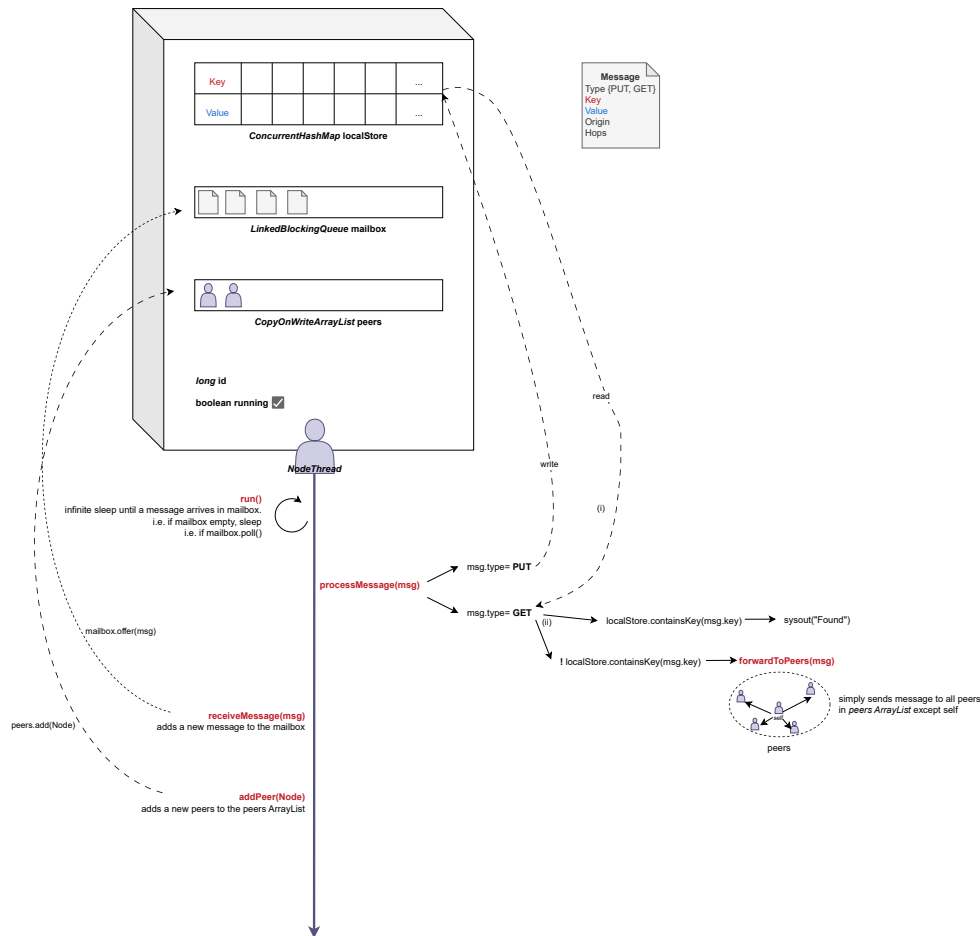
FIGURE 12 – Architecture interne et fonctionnement du NodeThread . Ce diagramme détaille la composition d'un nœud. La flèche verticale symbolise le thread actif, tandis que la boîte 3D représente l'objet Node avec son état ( id , running ) et ses structures ( peers , localStore ). La structure Message est dessinée en gris pour montrer qu'elle est stockée dans la mailbox . Les mots clés Key et Value sont mis en évidence pour montrer le transfert d'information du message vers le stockage local. Les fonctions principales sont aussi décrites : run() maintient le nœud actif, receiveMessage() ajoute les requêtes à la file, et processMessage() traite la logique métier.
