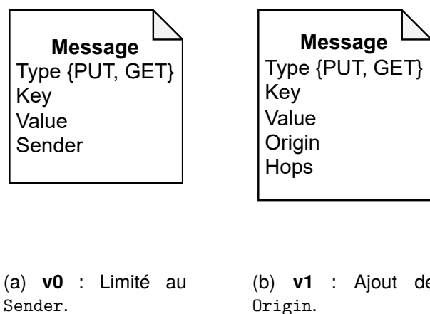
FIGURE 13 – Comparaison de l'évolution de la structure du Message.
