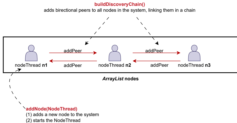
FIGURE 12 – Topologie et initialisation du réseau via DHTSystem. Ce schéma illustre l'organisation des nœuds stockés dans une ArrayList. En bas, la fonction addNode() est indiquée comme responsable de l'ajout d'un nouveau nœud et du démarrage de son thread. En haut, la fonction buildDiscoveryChain() est mise en évidence : elle parcourt la liste pour établir des connexions bidirectionnelles entre les nœuds voisins. Ces connexions sont matérialisées par les flèches rouges addPeer , transformant la simple liste en une chaîne de propagation opérationnelle.
