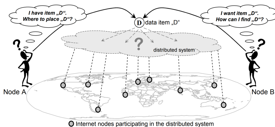
FIGURE 1 – Le problème du lookup : le nœud A stocke une donnée D et le nœud B doit la retrouver sans connaître son emplacement. [Source:schéma pris des notes de cours DBLP:conf/p2p/WehrleGR05]
