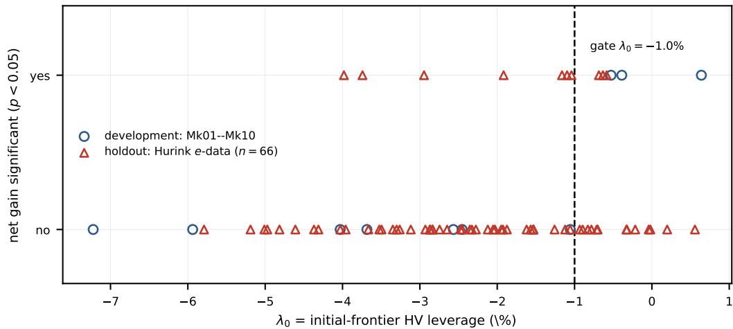
图 6: 零代门控的分离情况: 横轴为探针读数 \lambda_0 (初始前沿 HV 杠杆, %), 纵轴为“该实例的净增量是否显著为正”(是 = 上排, 否 = 下排), 每个标记是一个实例。虚线即门限 \lambda_0 = -1.0\% , 它在开发集(圆点)上标定后立即冻结, 再原样用到留出集(三角)上。门控理想的效果是“门限右侧全在上排、左侧全在下排”, 实际并非如此: 留出集在门限右侧仍有许多三角落在下排——被放行的实例里有相当一部分其实并不赚。
