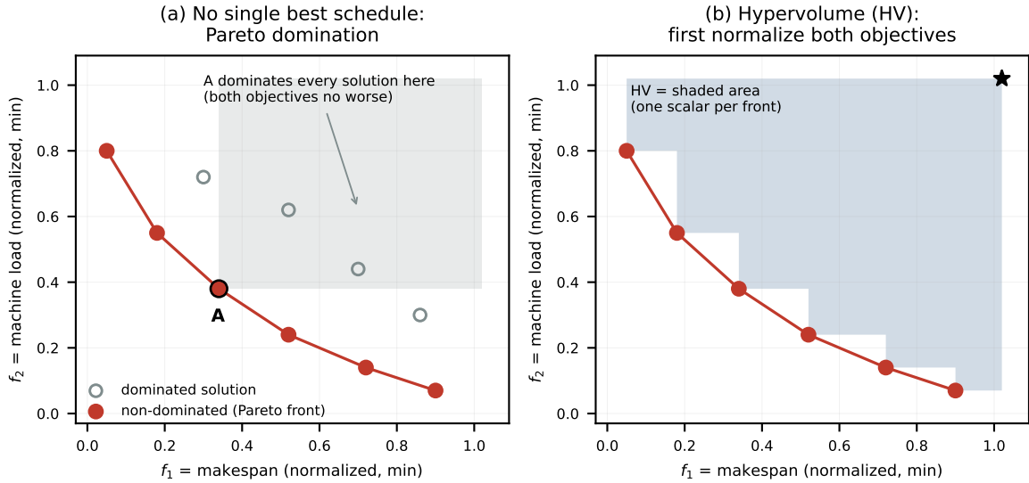
图 1: 概念示意图——点为手工构造，非实验结果，不参与本文任何结论。(a) Pareto 支配：解 A 的两个目标都不差于阴影区内任何解，故那些解“被 A 支配”；互不支配的解（红）连成 Pareto 前沿。(b) 超体积 HV：双目标要先归一化（两轴各自缩放到 [lo, hi] ），HV 才等于前沿与参考点之间围出的面积；而 lo/hi 如何取定正是 §4 的主题。
