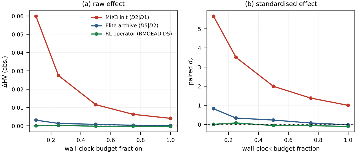
图 4: 算力-算法响应面。(a) 原始 \Delta HV 随墙钟预算的衰减; (b) 标准化效应 d_z 。初始化 (红) 是唯一随算力增加而衰减的显著效应, RL 选算子 (绿) 全程贴零。
