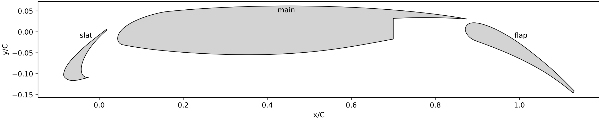
Official HLPW4 30P30N geometry: actual numerical wall contours
