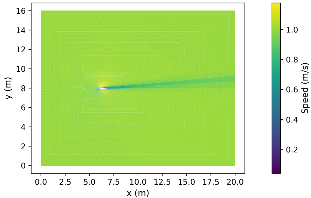
naca 128x52
