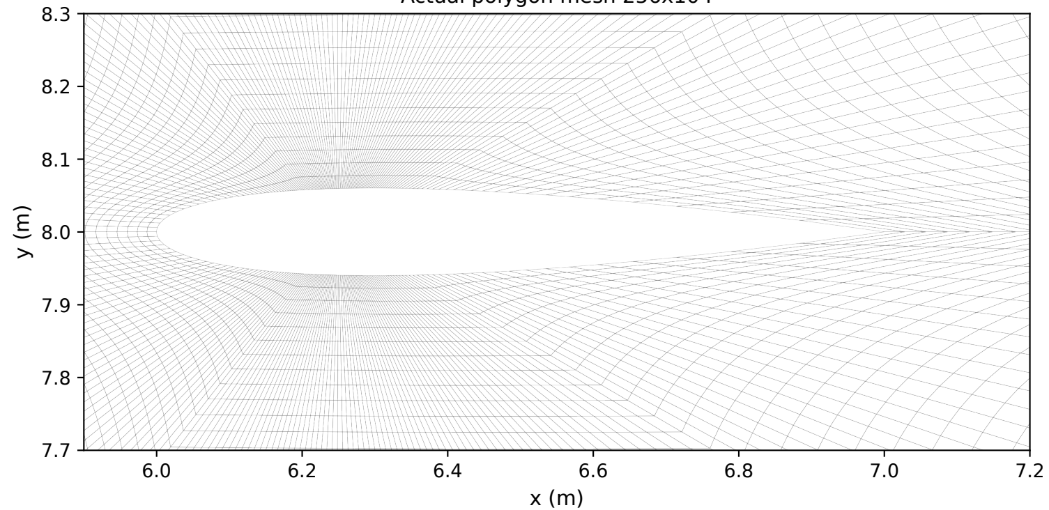
Actual polygon mesh 256x104
