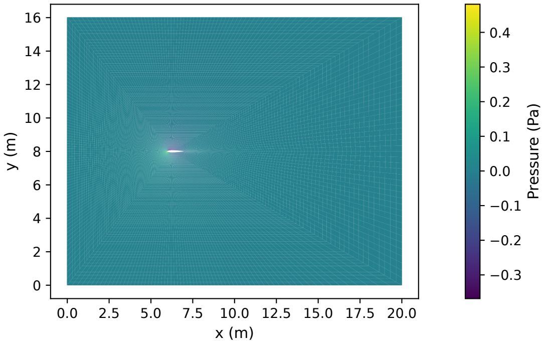
naca 256x104
