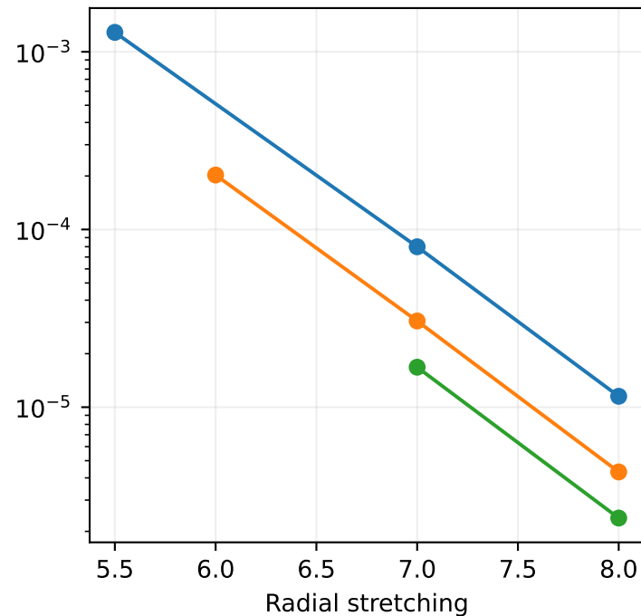
Initial explicit diffusion dt ceiling
