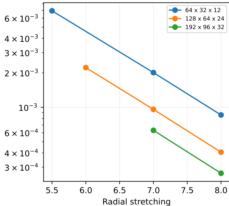
Actual maximum wall distance / D
