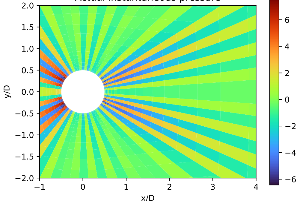
Actual instantaneous pressure
