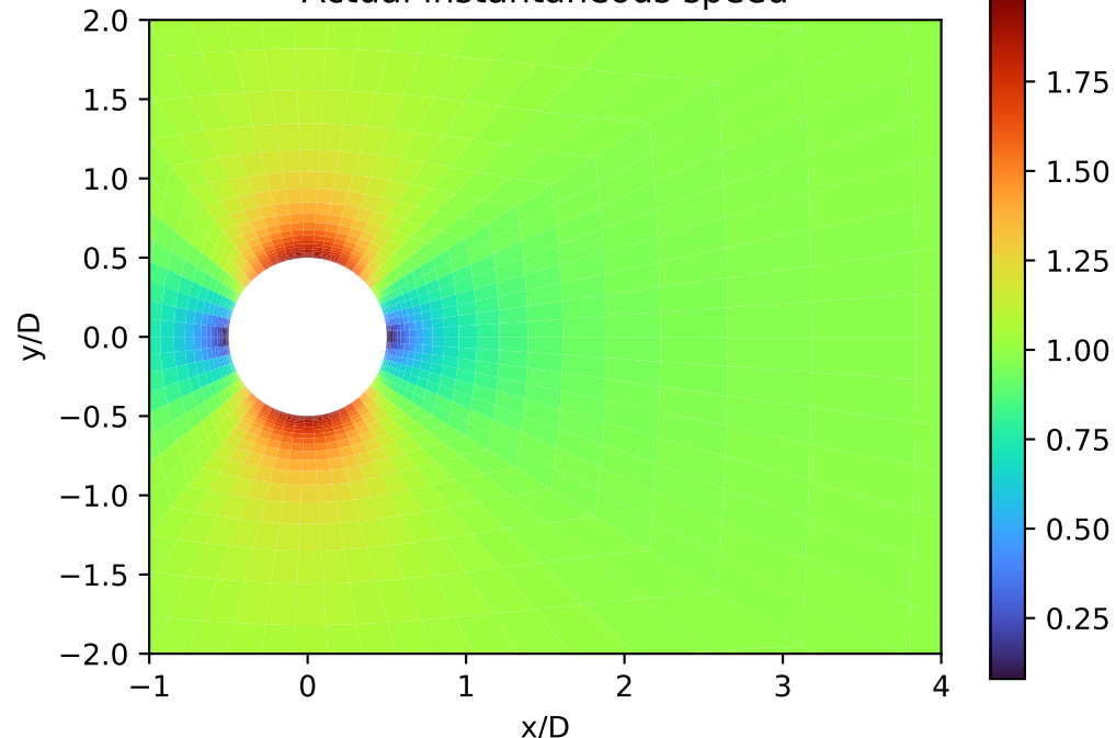
Actual instantaneous speed
