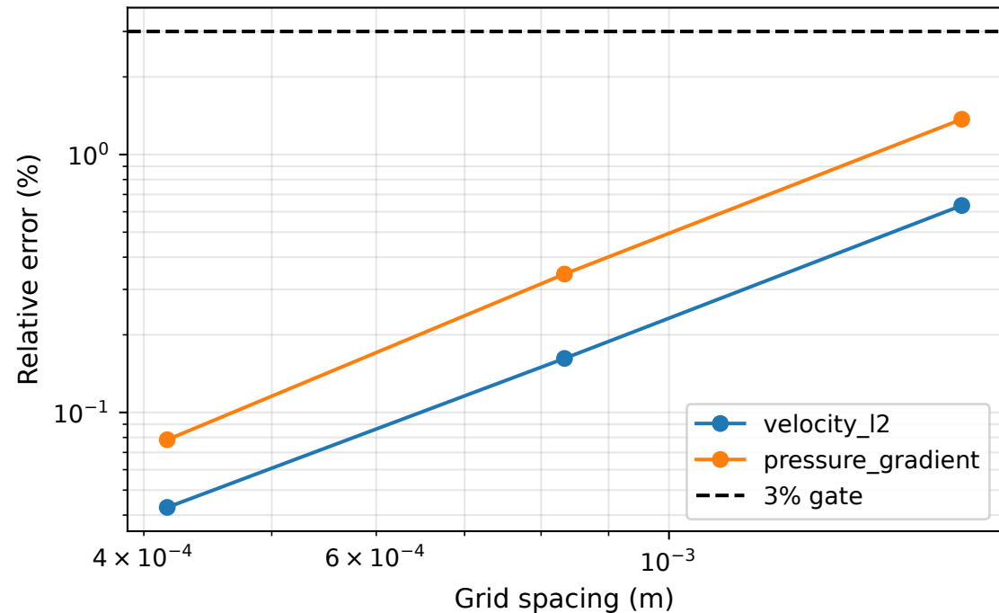
poiseuille: spatial refinement
