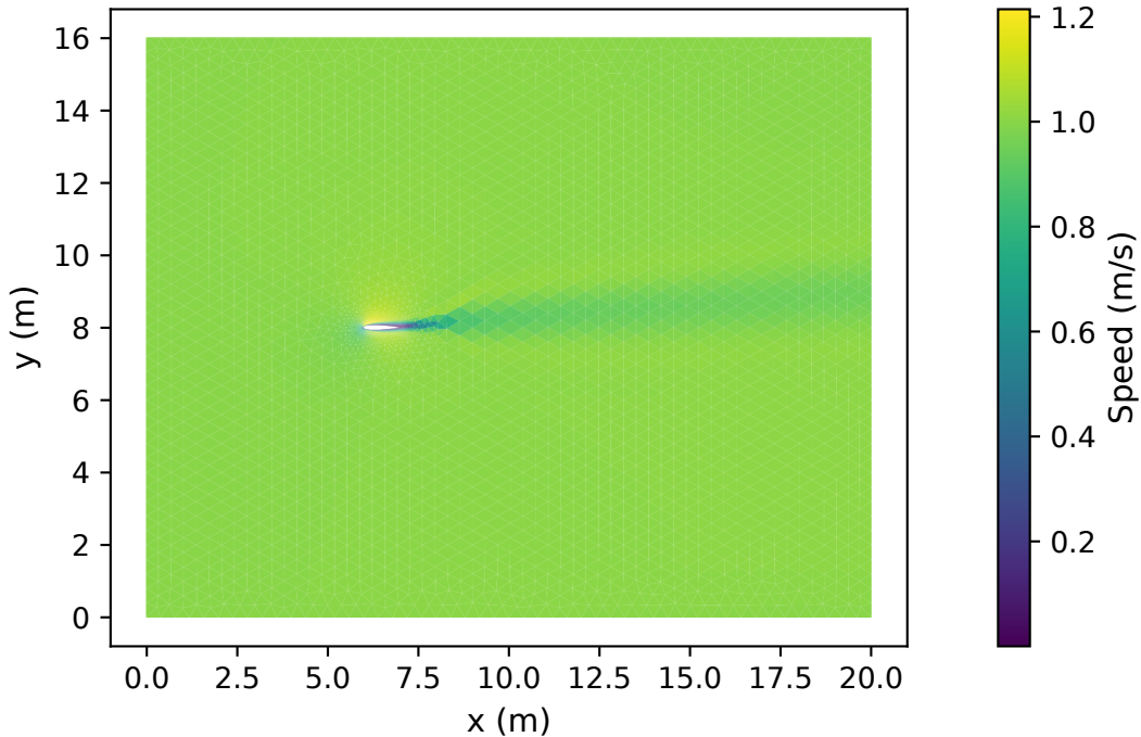
naca: 15018 cells
