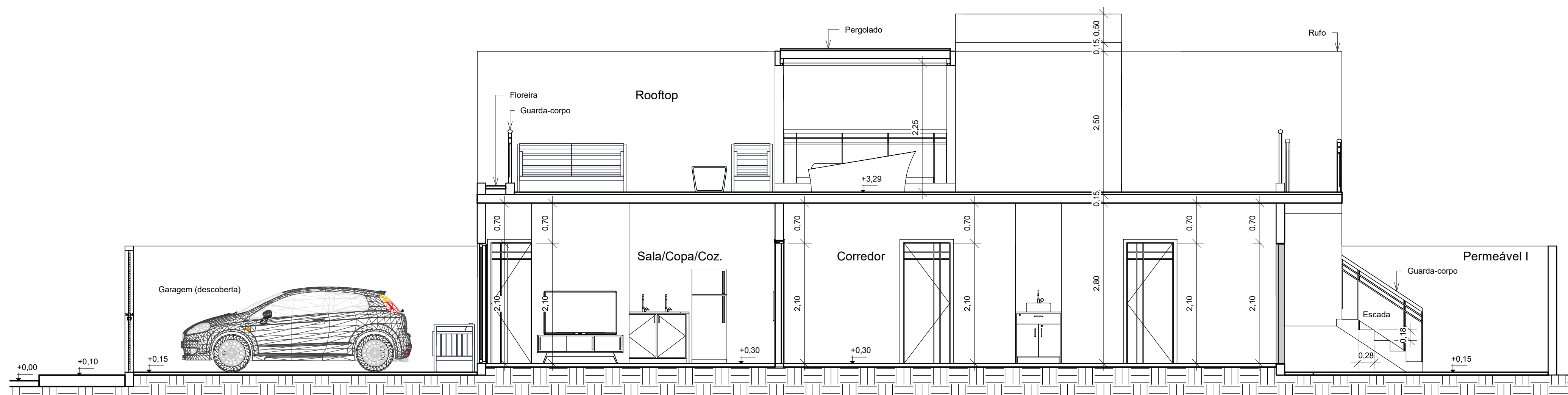
3 Corte A-A 1 : 50
