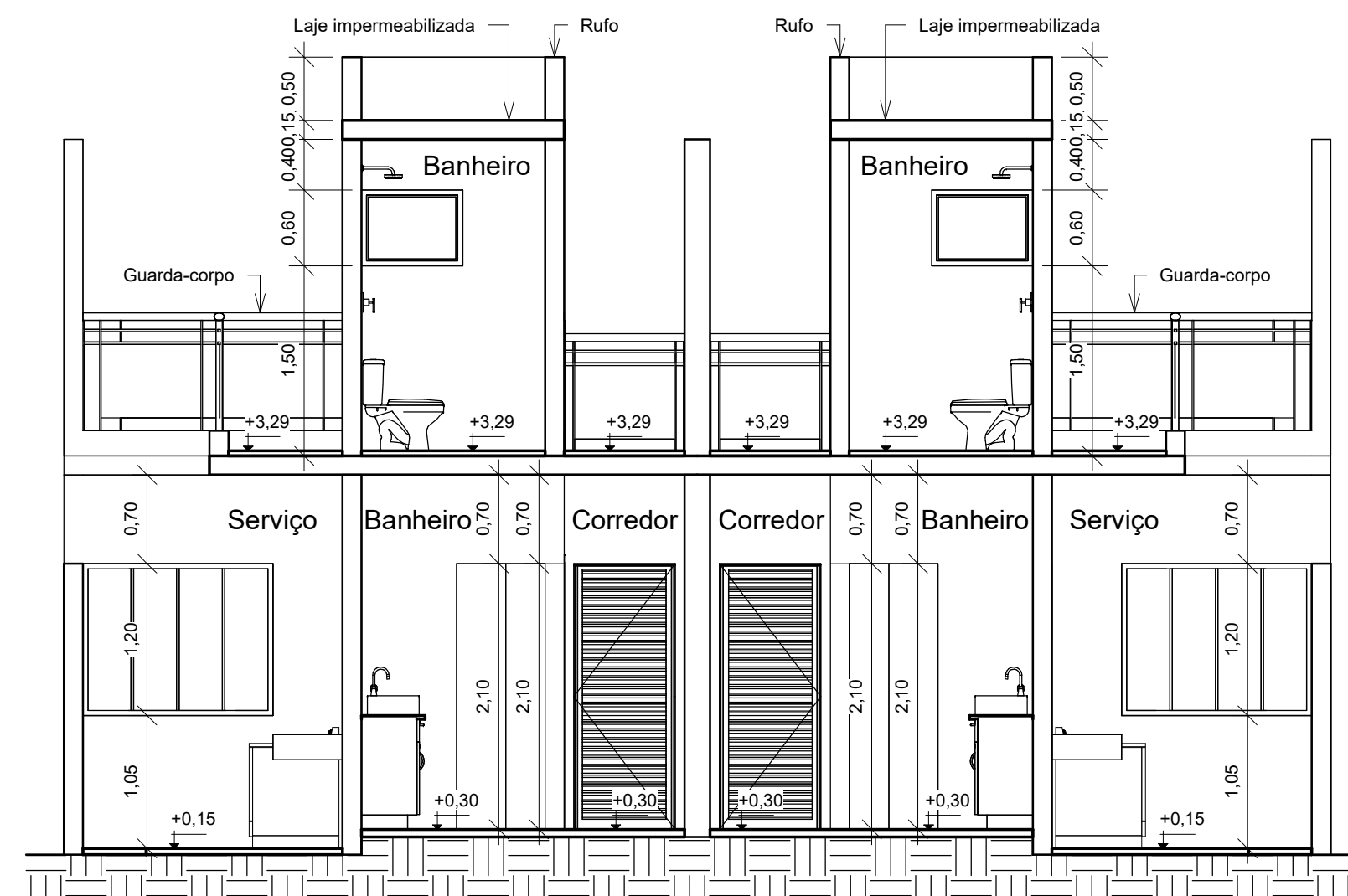
4 Corte B-B 1 : 50
