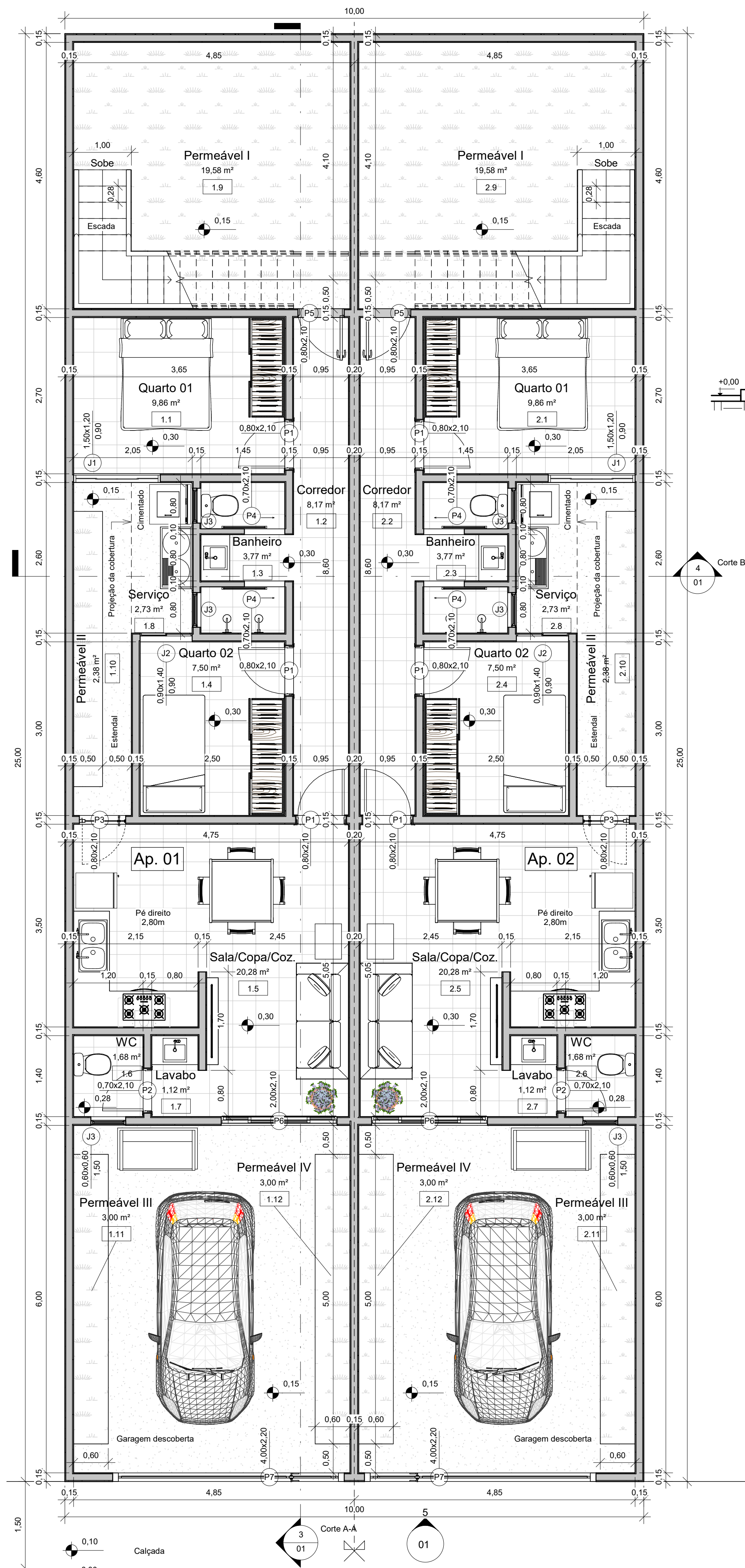
1 Pav. Térreo 1 : 50
