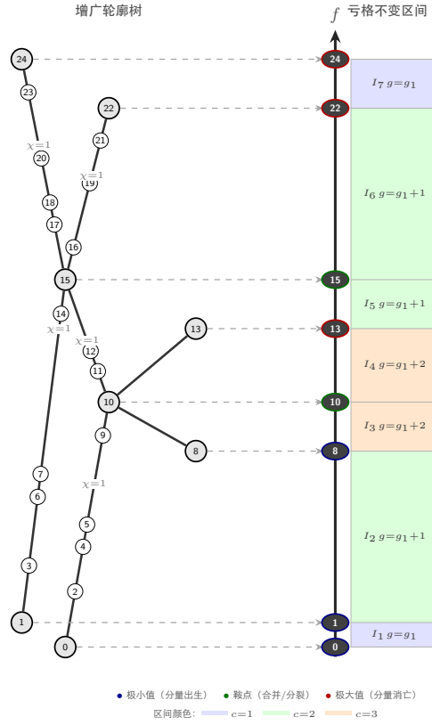
图 2: 增广轮廓树与亏格不变区间。左: 增广轮廓树 (灰色圆为结构节点, 白色圆为普通节点); 右: 临界点投影到标量轴后划分出的亏格不变区间 I_1 – I_7 (颜色表示连通分量数 c , 各区间内亏格 g 保持不变)。
