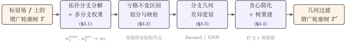
图 1: 方法整体流程。输入增广轮廓树经拓扑分支分解、亏格不变区间划分、分支几何差异计算后，由贪心算法筛选保留节点并重建简化树。
