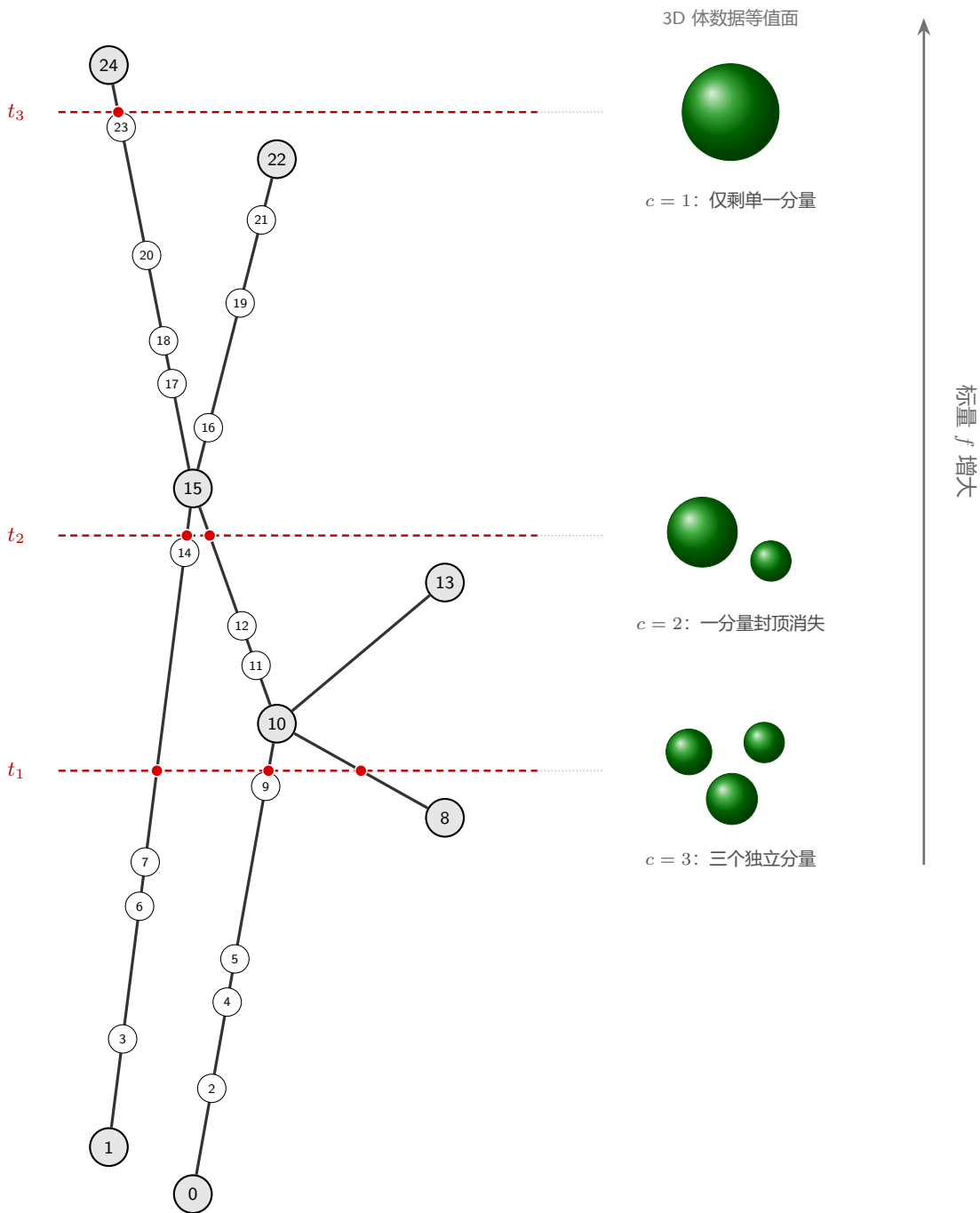
增广轮廓树与等值面连通性 ( c: 3 \rightarrow 2 \rightarrow 1 )
